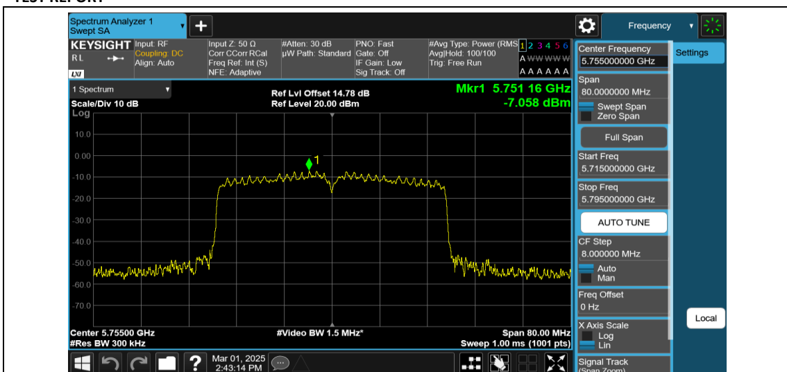
11AX40MIMO-Ant1-5755-PASS
