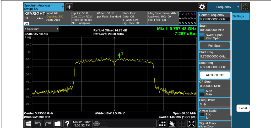
11AX40MIMO-Ant1-5795-PASS
