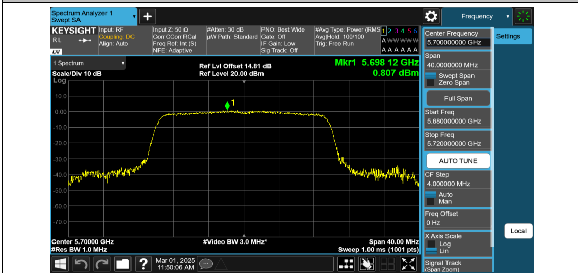
11AX20MIMO-Ant1-5700-PASS
