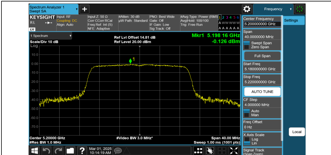
11AX20MIMO-Ant1-5200-PASS
