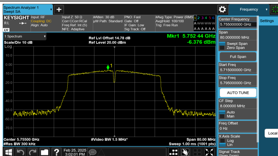
11N40MIMO-Ant1-5755-PASS
