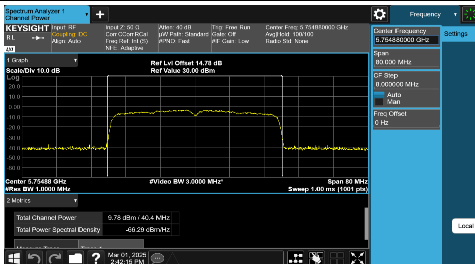
11AX40MIMO-Ant1-5755-PASS
