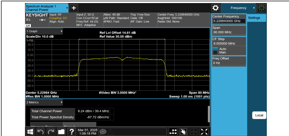
11AX40MIMO-Ant1-5230-PASS
