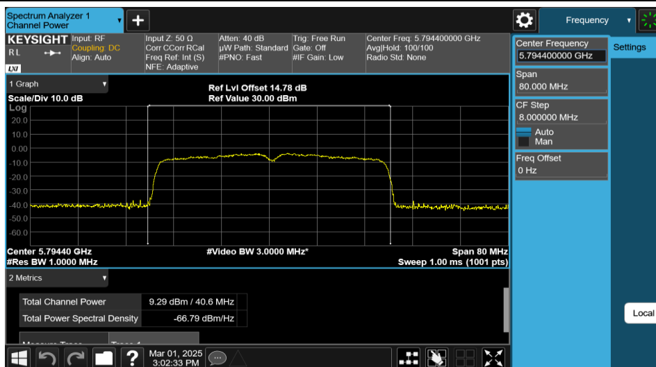
11AX40MIMO-Ant1-5795-PASS
