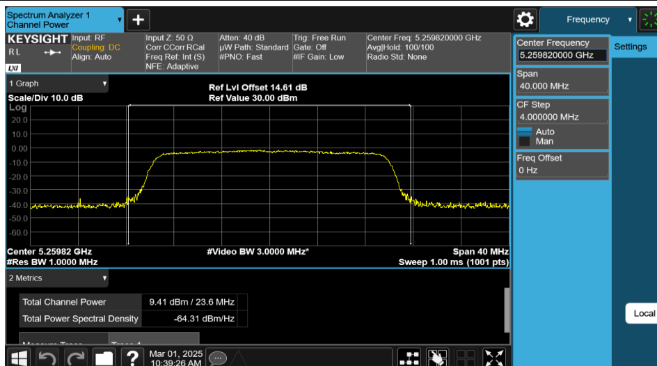
11AX20MIMO-Ant1-5260-PASS
