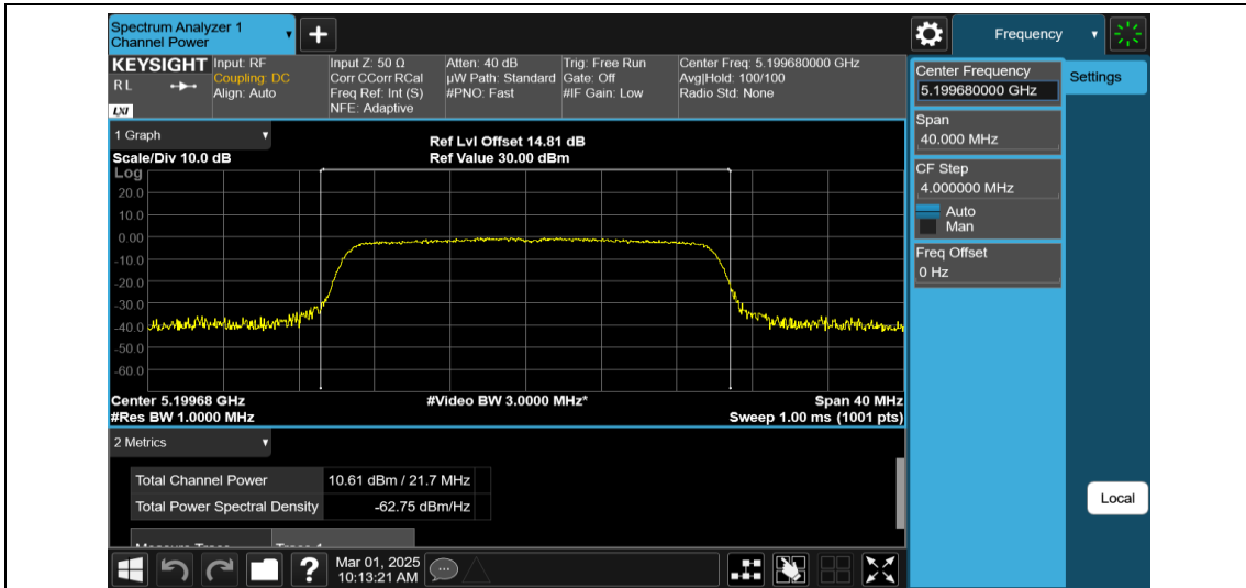
11AX20MIMO-Ant1-5200-PASS
