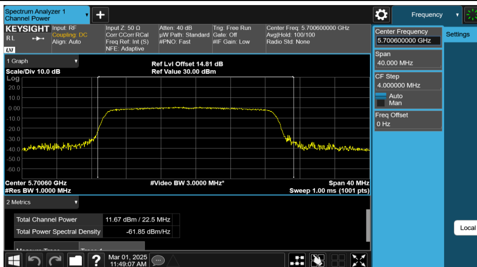
11AX20MIMO-Ant1-5700-PASS
