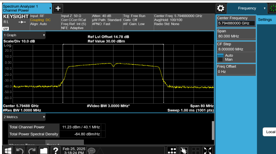
11N40MIMO-Ant1-5795-PASS
