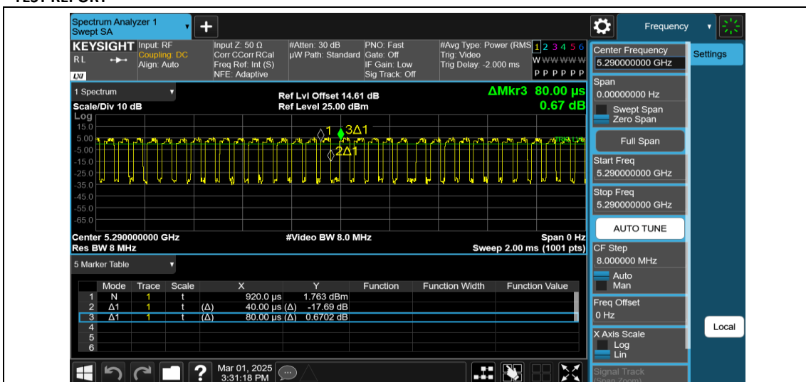
NTNV-11AX80MIMO-Ant1-5290
