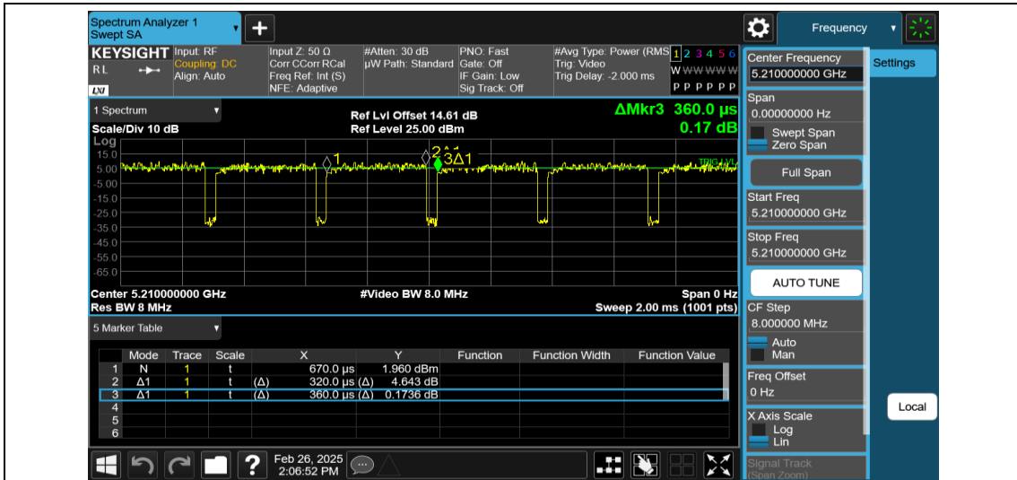
NTNV-11AC80MIMO-Ant1-5210
