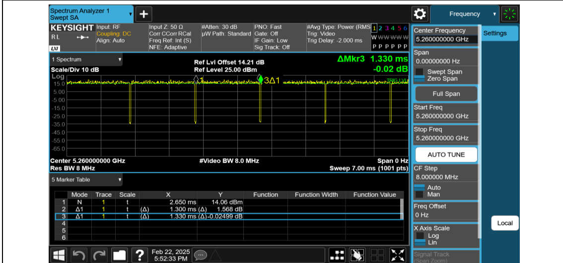
NTNV-11N20MIMO-Ant2-5260
