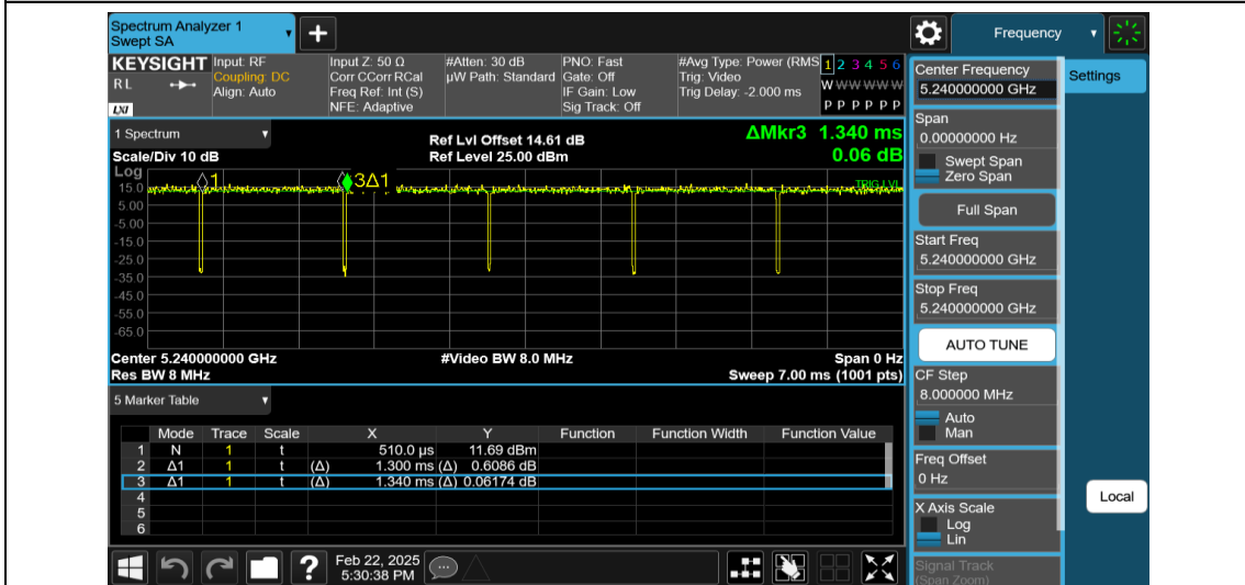
NTNV-11N20MIMO-Ant1-5240
