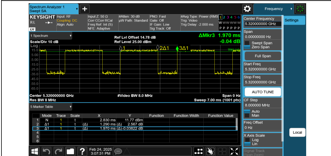
NTNV-11N20MIMO-Ant1-5320
