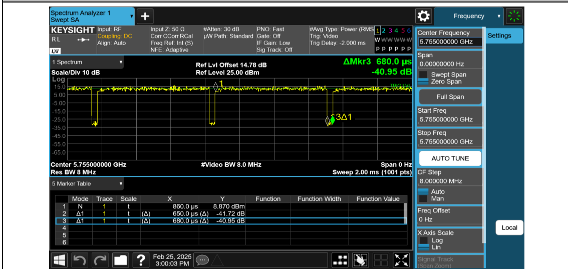
NTNV-11N40MIMO-Ant1-5755
