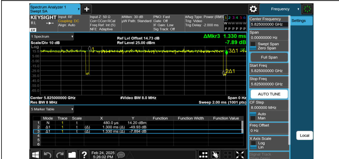
NTNV-11N20MIMO-Ant1-5825
