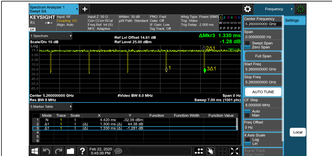
NTNV-11N20MIMO-Ant1-5260
