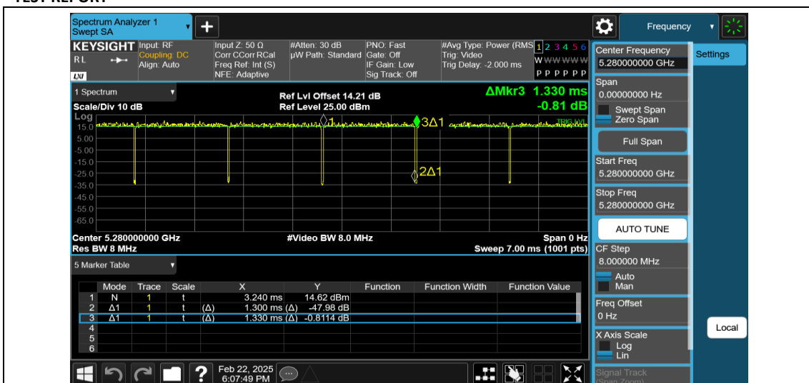
NTNV-11N20MIMO-Ant2-5280
