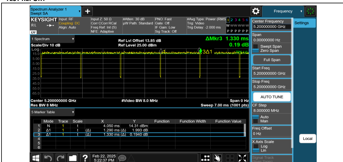
NTNV-11N20MIMO-Ant2-5200
