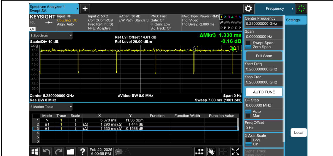
NTNV-11N20MIMO-Ant1-5280
