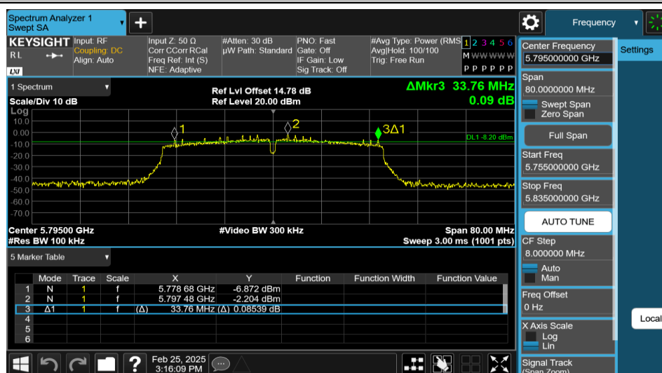
11N40MIMO-Ant1-5795-PASS
