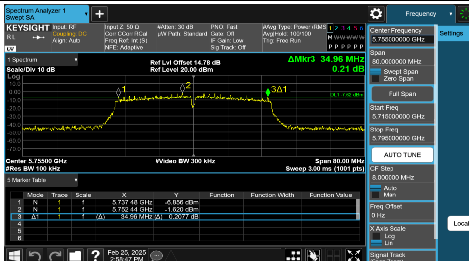
11N40MIMO-Ant1-5755-PASS
