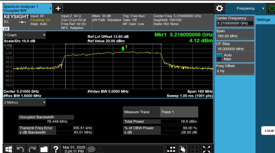
11AX80MIMO-Ant2-5210
