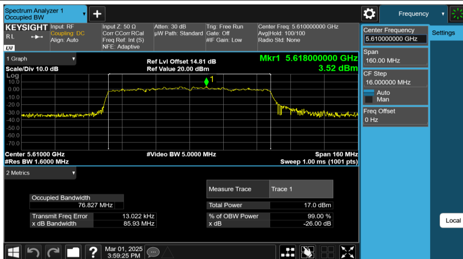
11AX80MIMO-Ant1-5610
