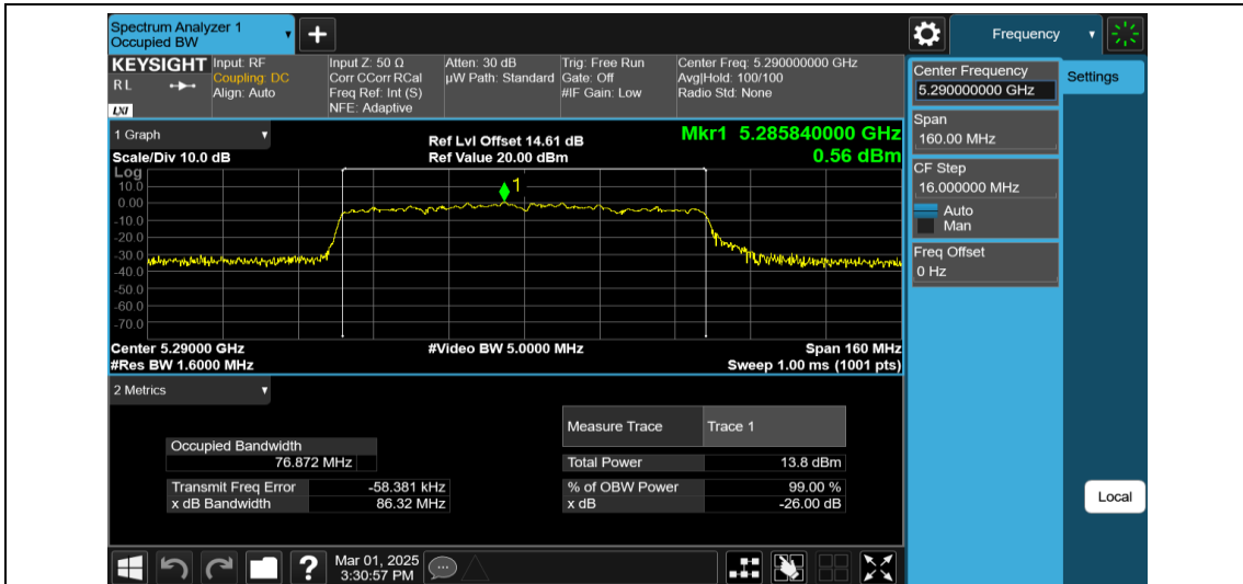
11AX80MIMO-Ant1-5290
