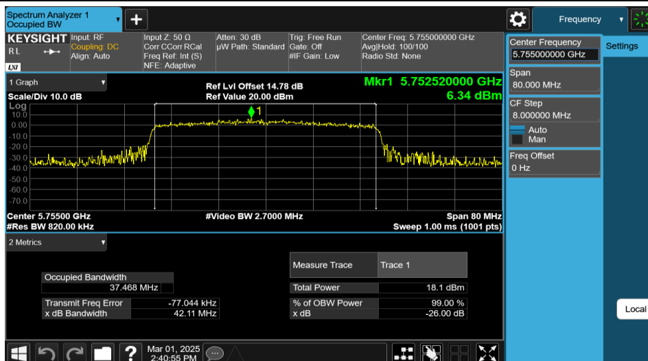
11AX40MIMO-Ant1-5755
