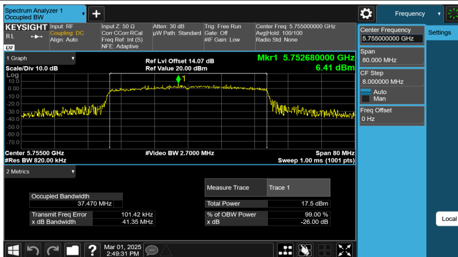
11AX40MIMO-Ant2-5755
