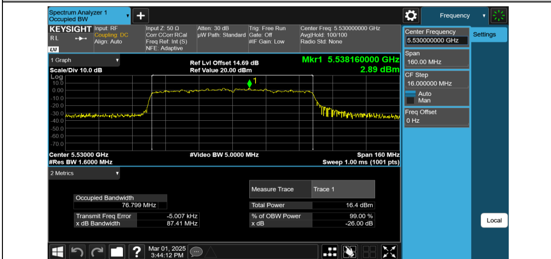
11AX80MIMO-Ant1-5530
