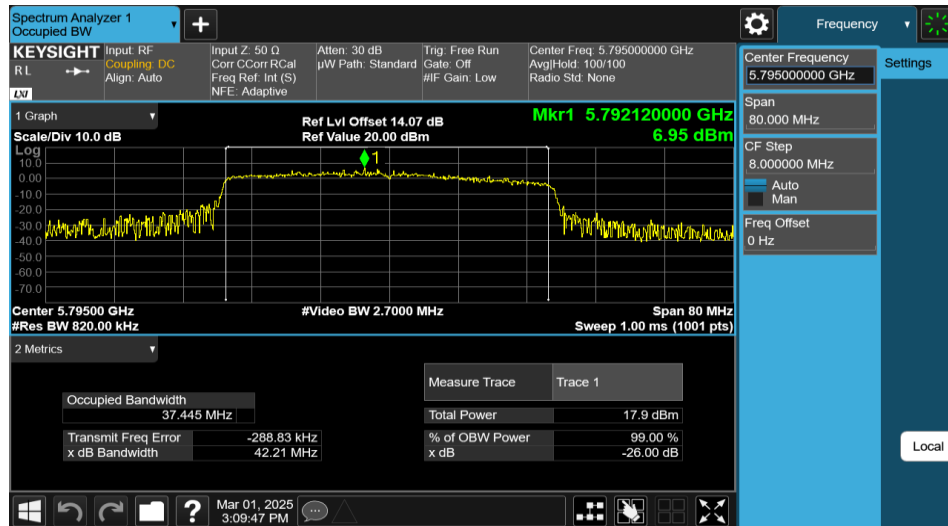
11AX40MIMO-Ant2-5795
