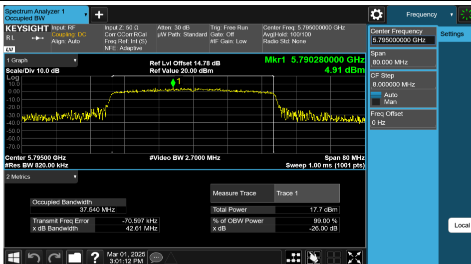
11AX40MIMO-Ant1-5795
