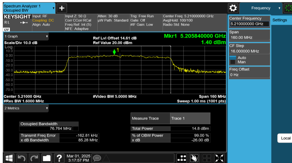
11AX80MIMO-Ant1-5210
