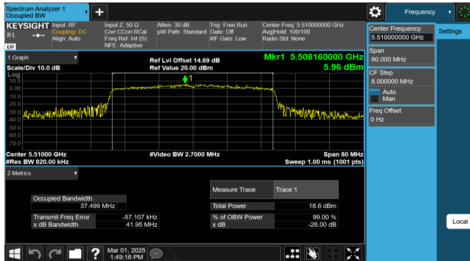
11AX40MIMO-Ant1-5510
