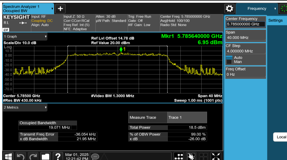
11AX20MIMO-Ant1-5785
