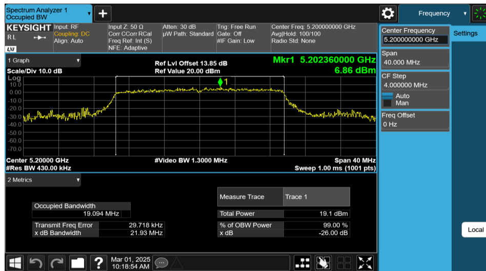
11AX20MIMO-Ant2-5200
