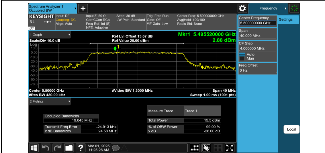
11AX20MIMO-Ant2-5500
