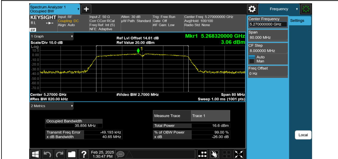
11N40MIMO-Ant1-5270
