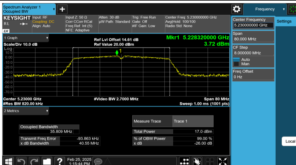
11N40MIMO-Ant1-5230
