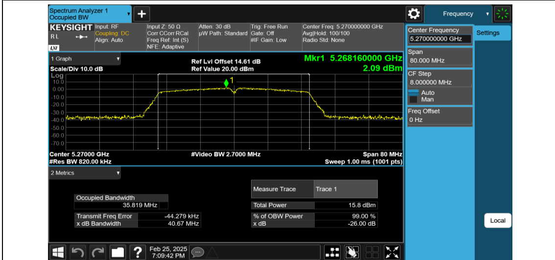
11AC40MIMO-Ant1-5270
