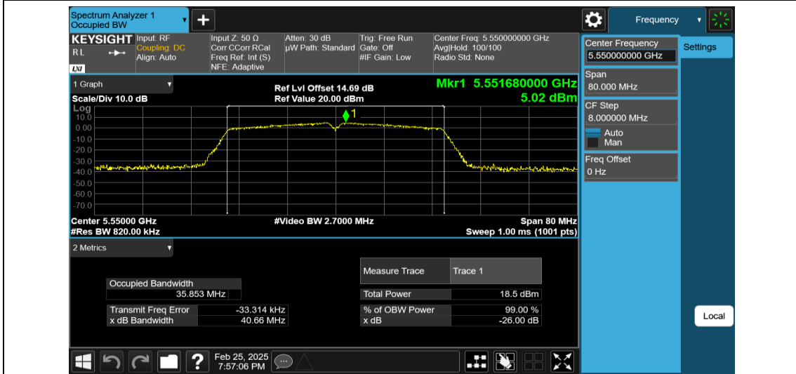
11AC40MIMO-Ant1-5550
