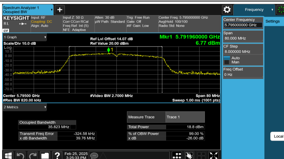
11N40MIMO-Ant2-5795
