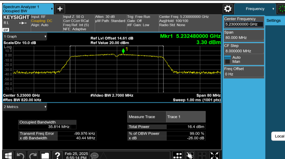
11AC40MIMO-Ant1-5230
