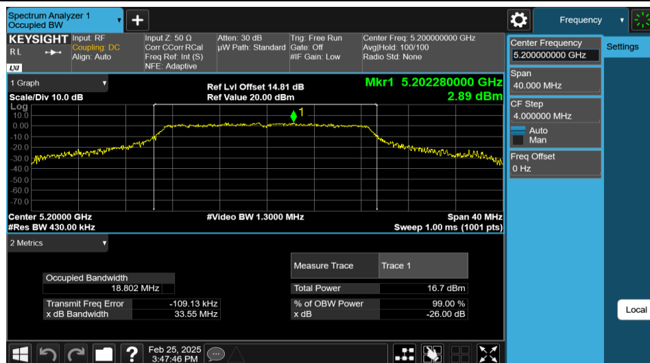
11AC20MIMO-Ant1-5200
