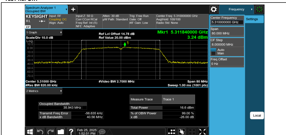
11N40MIMO-Ant1-5310
