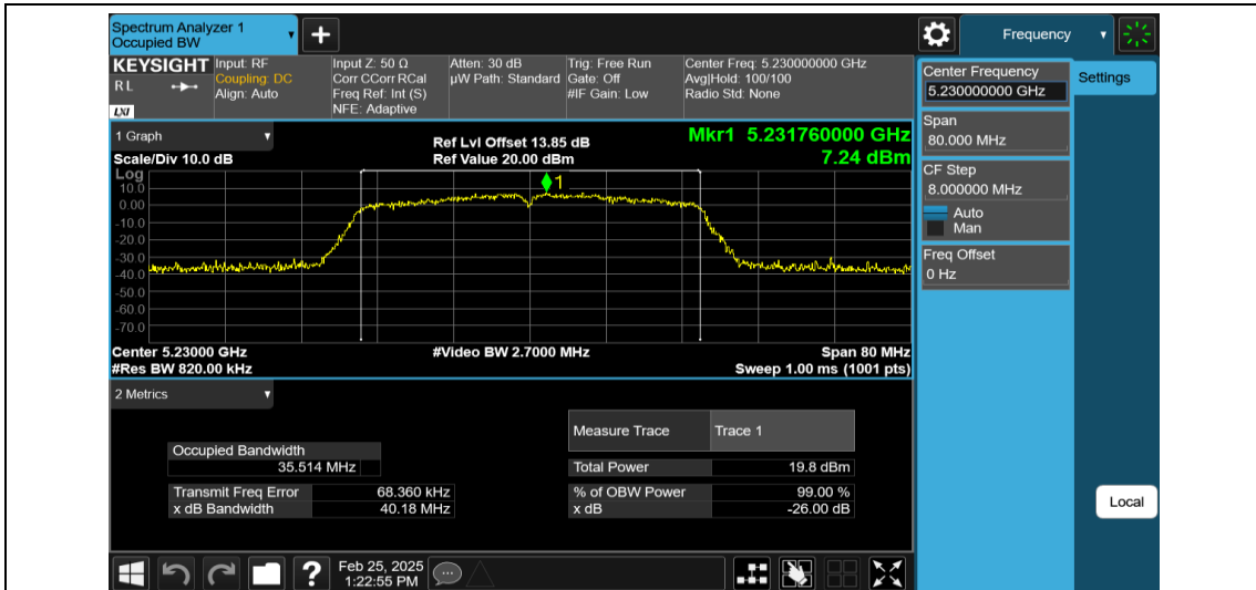
11N40MIMO-Ant2-5230
