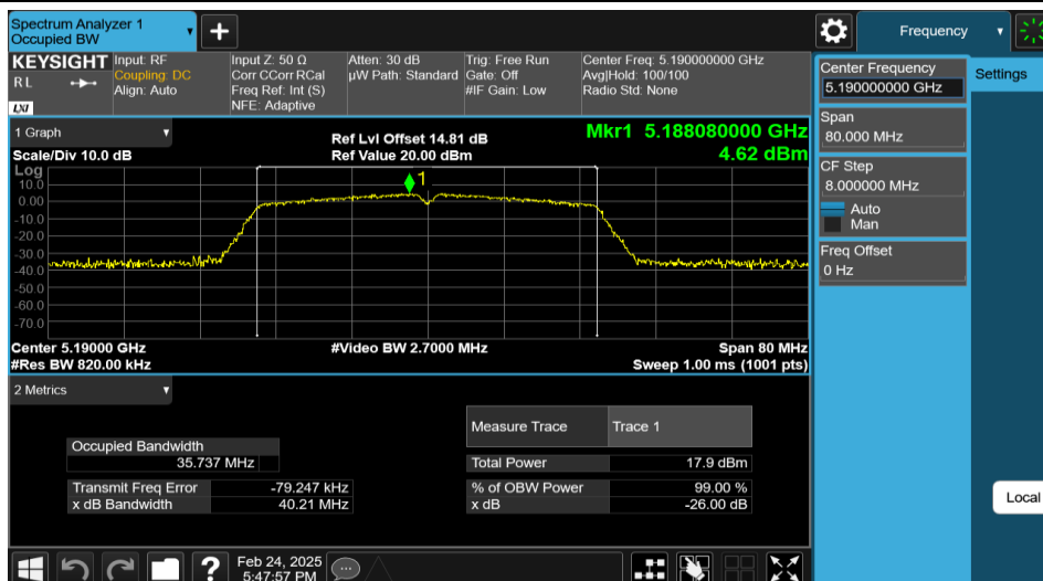
11N40MIMO-Ant1-5190
