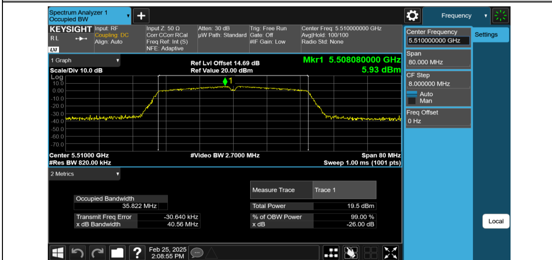
11N40MIMO-Ant1-5510
