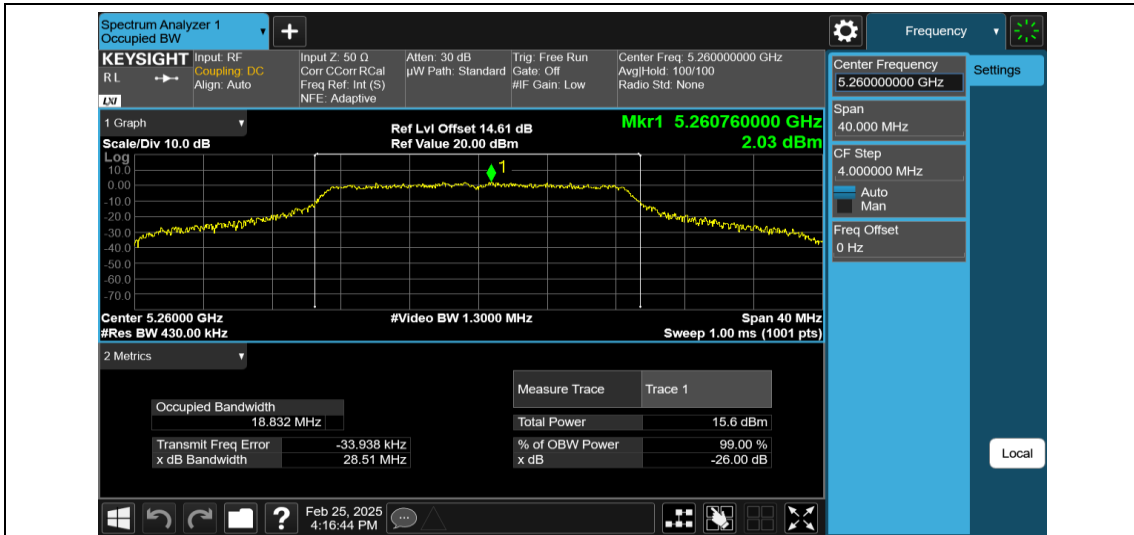
11AC20MIMO-Ant1-5260
