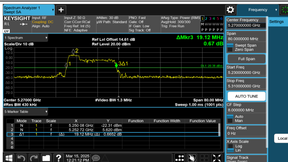
11AX40MIMO-Ant1-5270-52Tone-RU37
