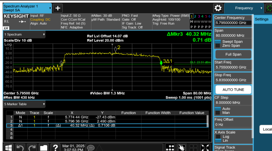
11AX40MIMO-Ant2-5795
