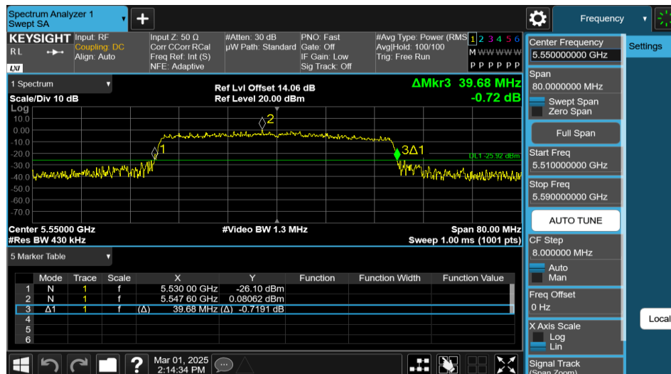
11AX40MIMO-Ant2-5550
