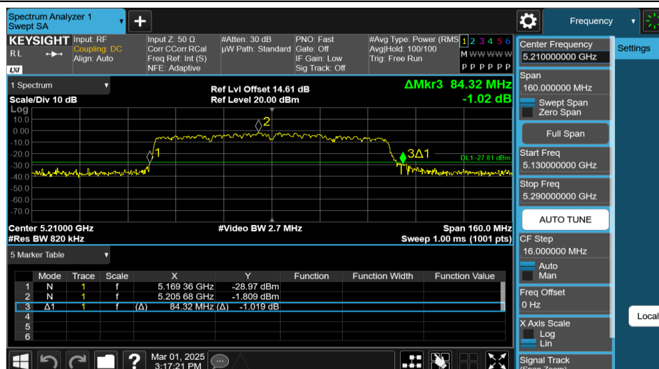
11AX80MIMO-Ant1-5210
