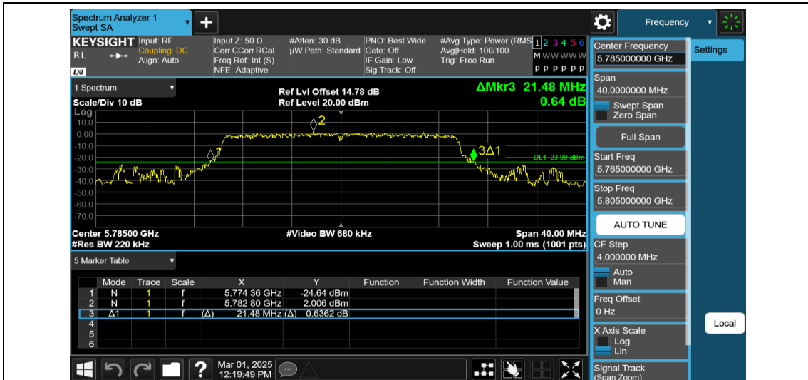
11AX20MIMO-Ant1-5785
