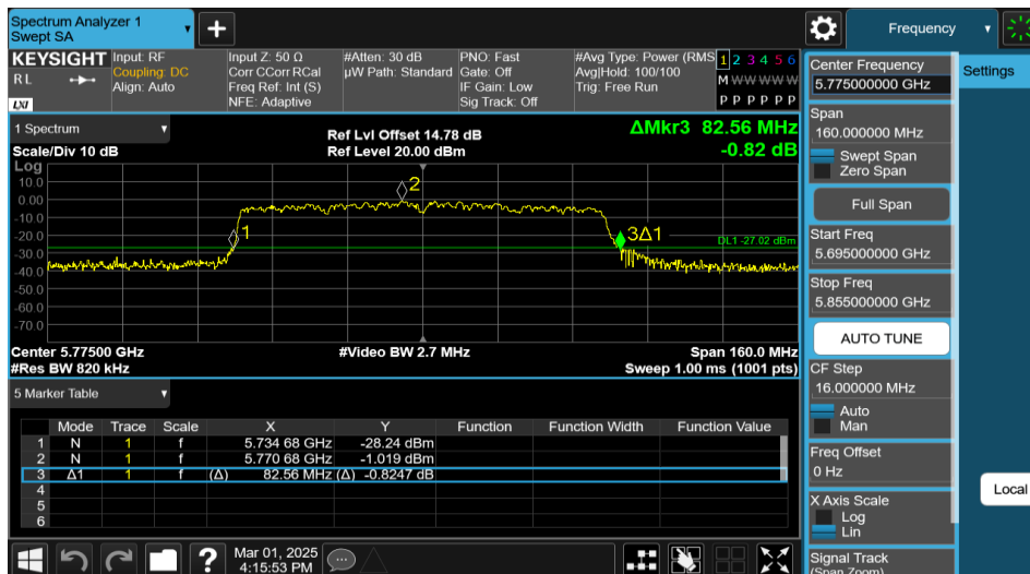
11AX80MIMO-Ant1-5775
