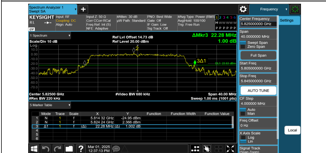
11AX20MIMO-Ant1-5825
