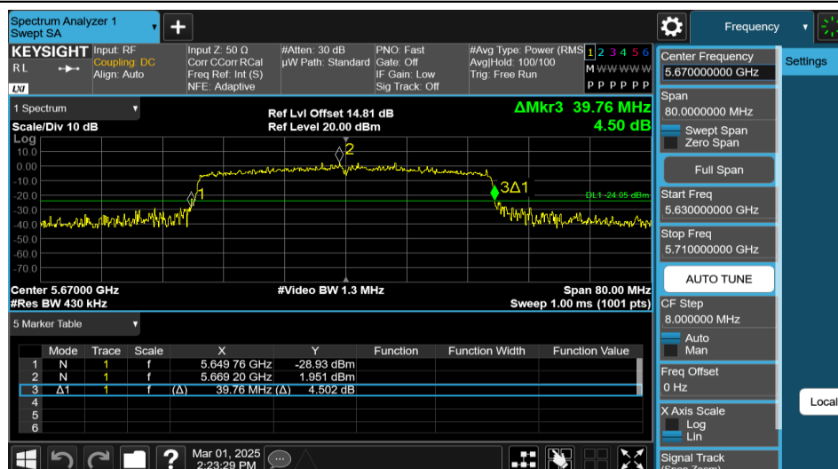
11AX40MIMO-Ant1-5670
