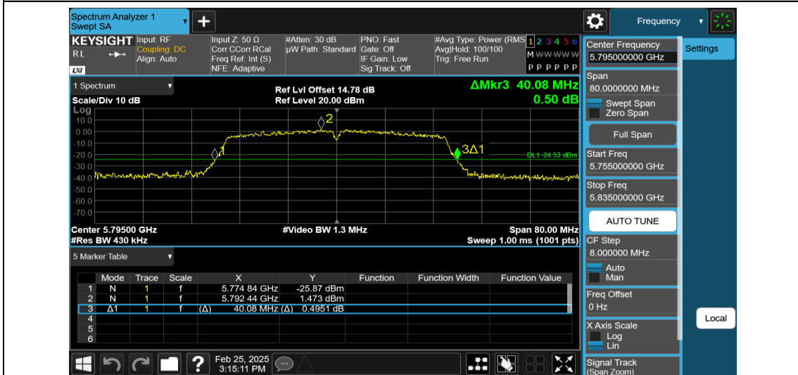
11N40MIMO-Ant1-5795
