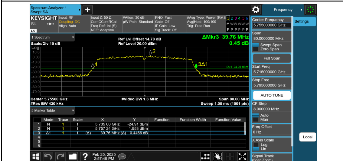
11N40MIMO-Ant1-5755
