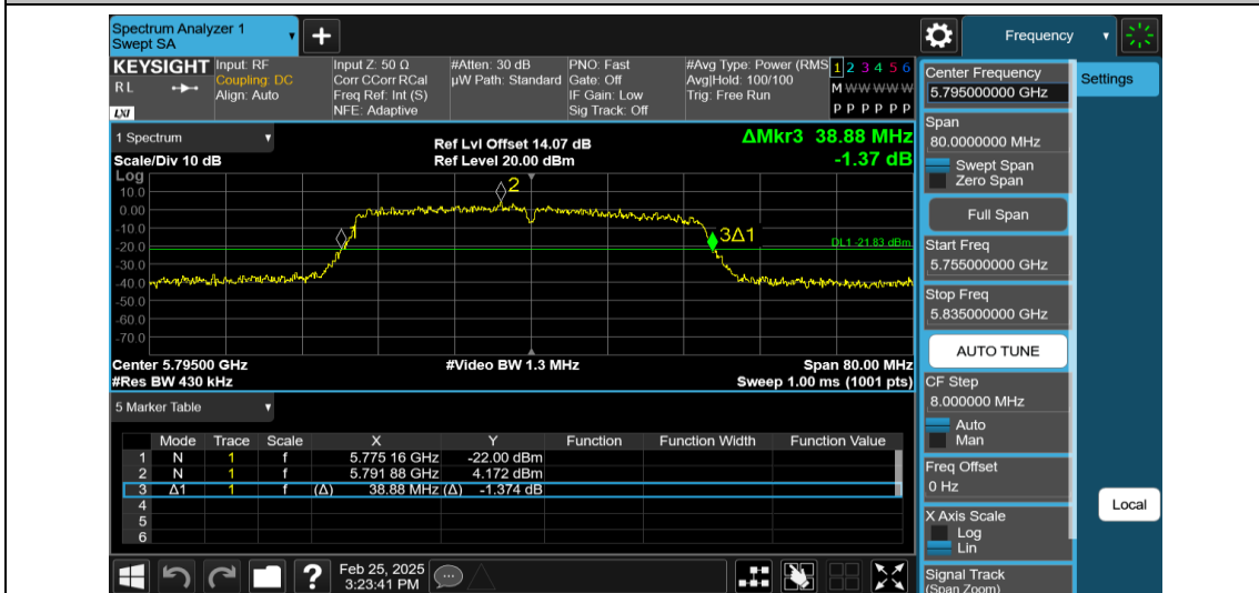
11N40MIMO-Ant2-5795
