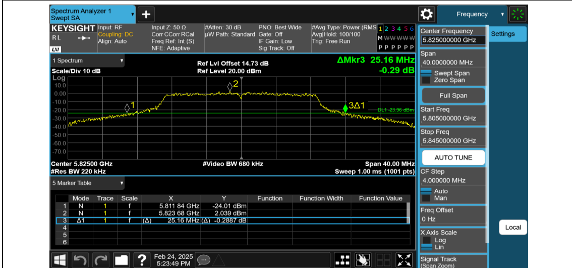
11N20MIMO-Ant1-5825
