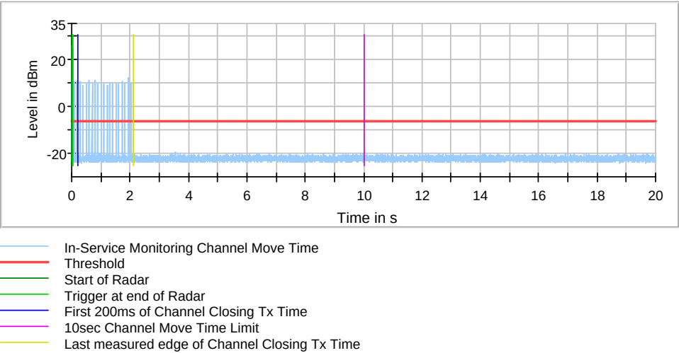
802.11n HT40 5270MHz
