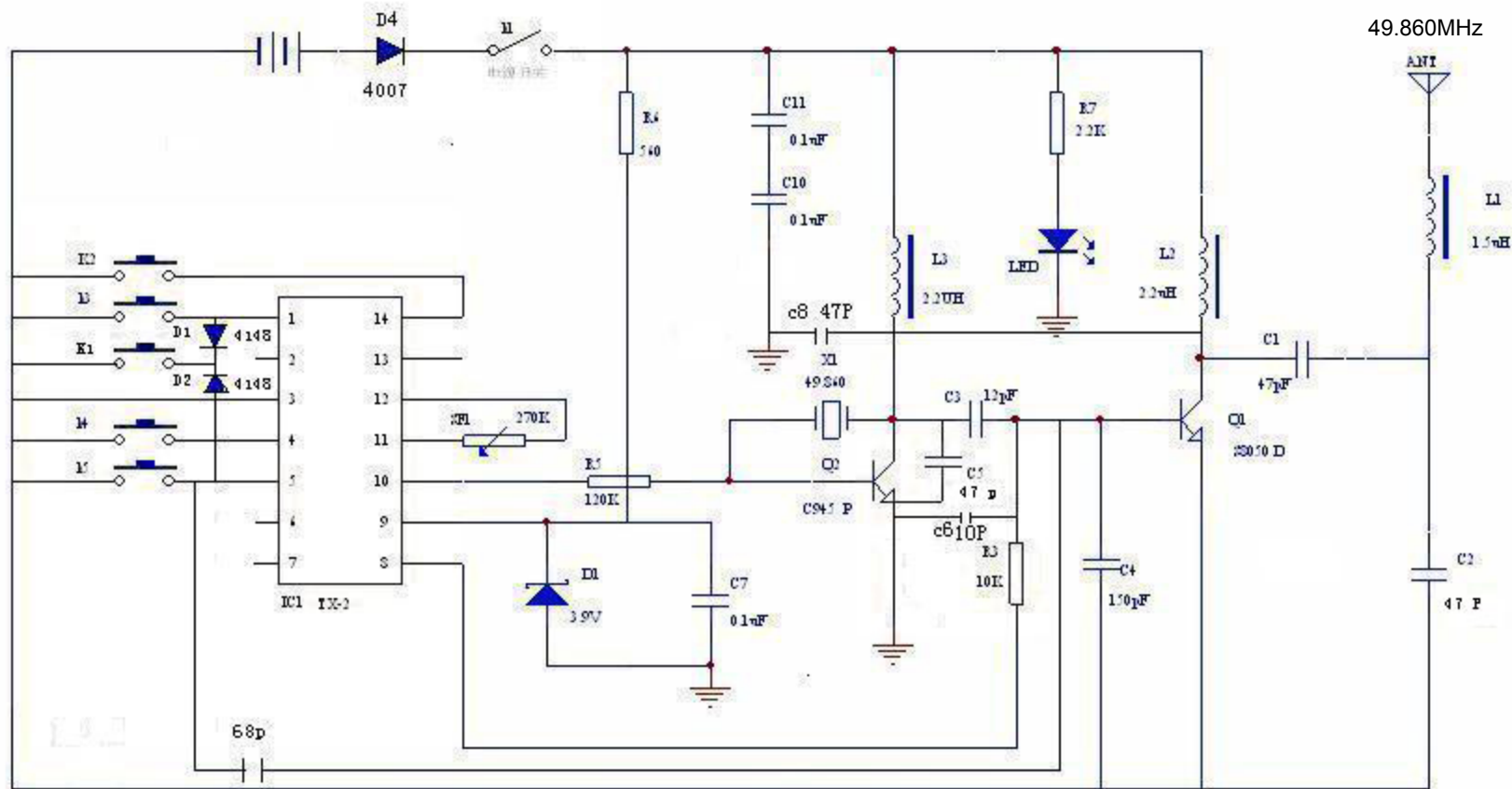
49.860M发射电路图
