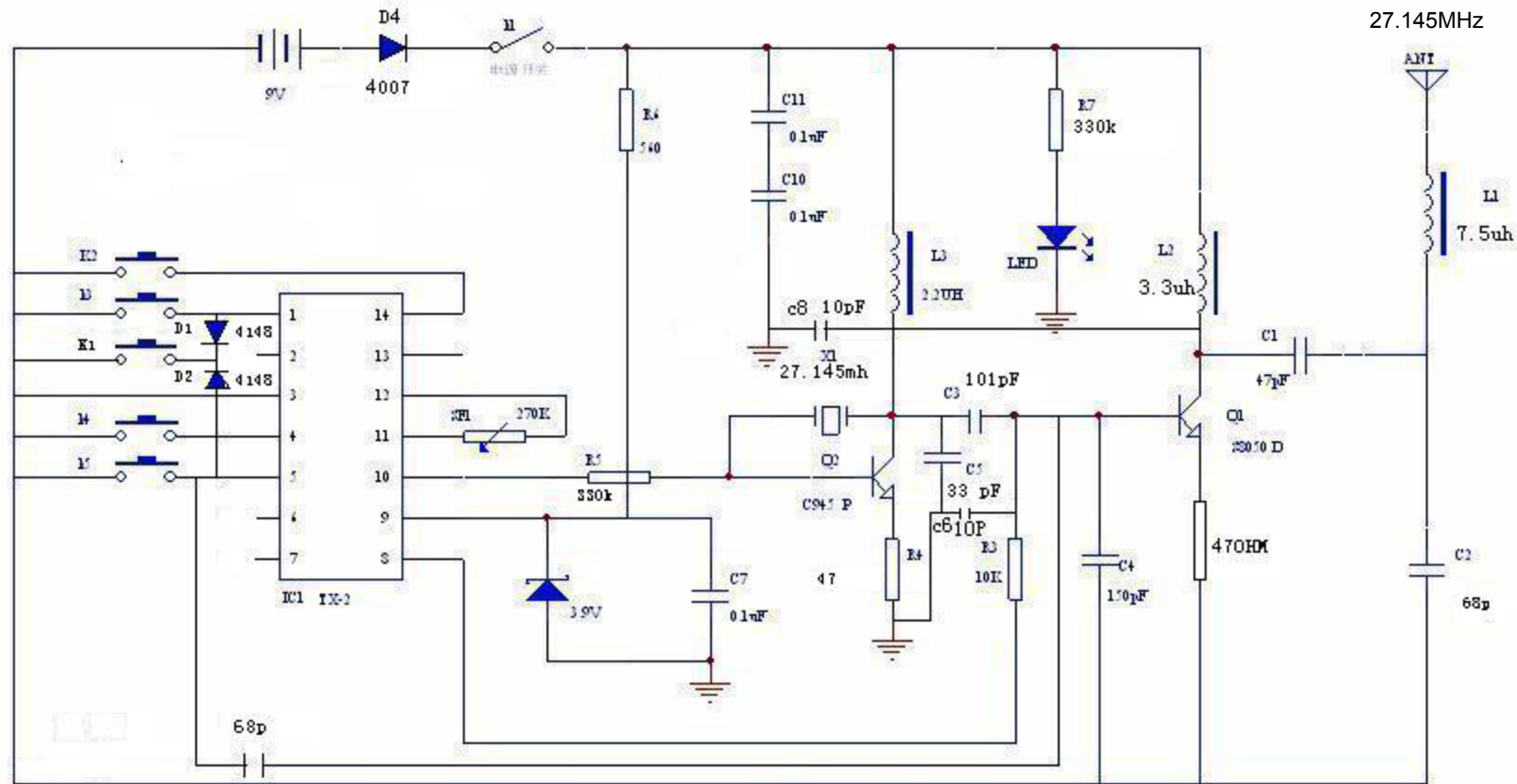
27.145 发射电路图
