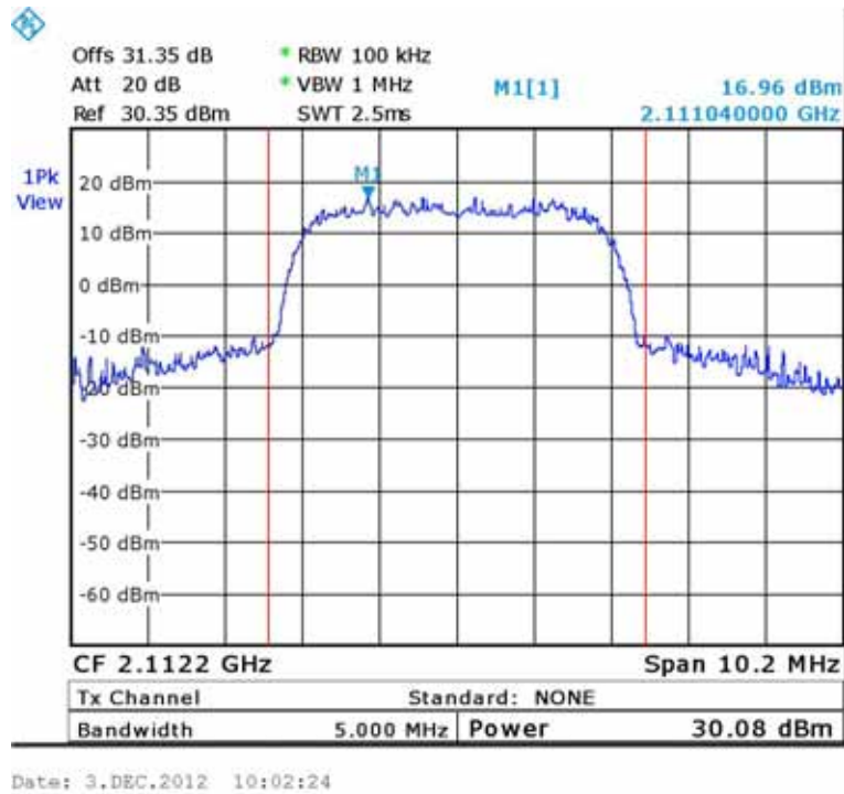
Figure 254.— W-CDMA (2112.2 MHz)
