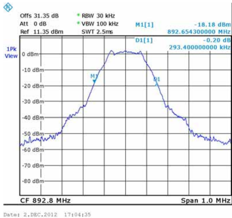
Figure 44.— Input 892.8 MHz.
