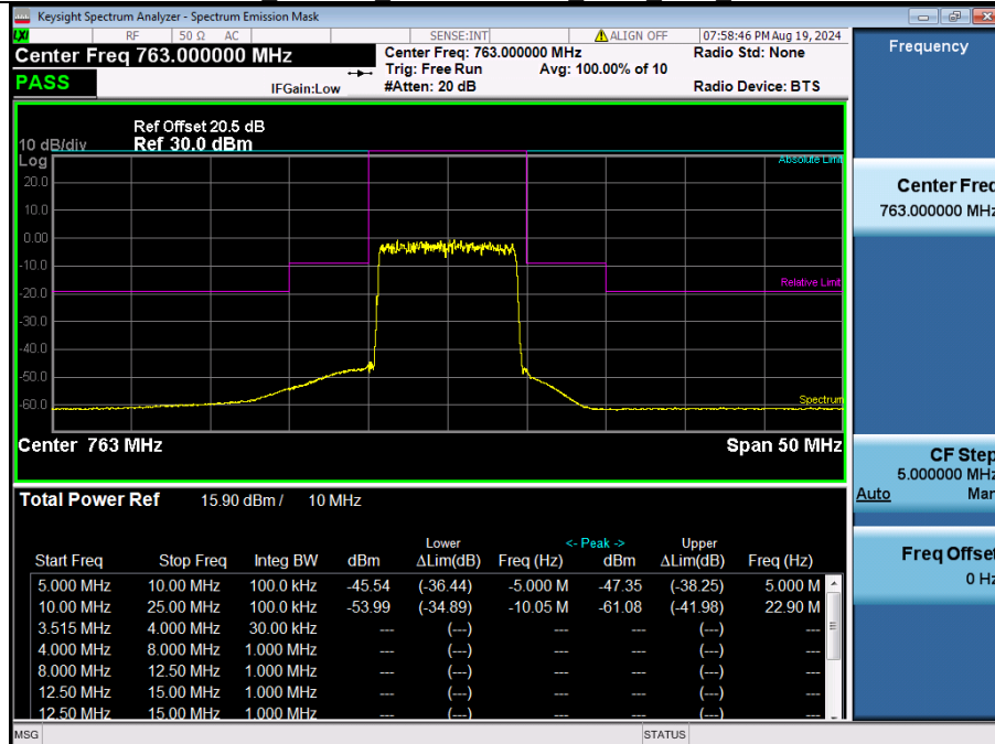
N14 763MHz AWGN-AGC+3 SISO Ant1 NTN
