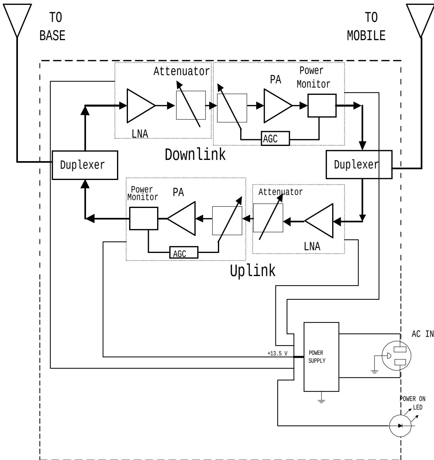
CBDA-ESMR-10W80-A ELECTRICAL SCHEMATICS
