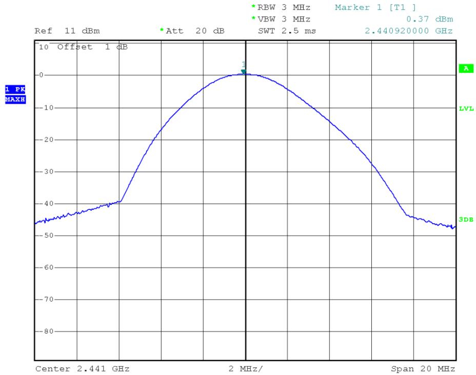
Plot B2: \pi/4 -DQPSK
