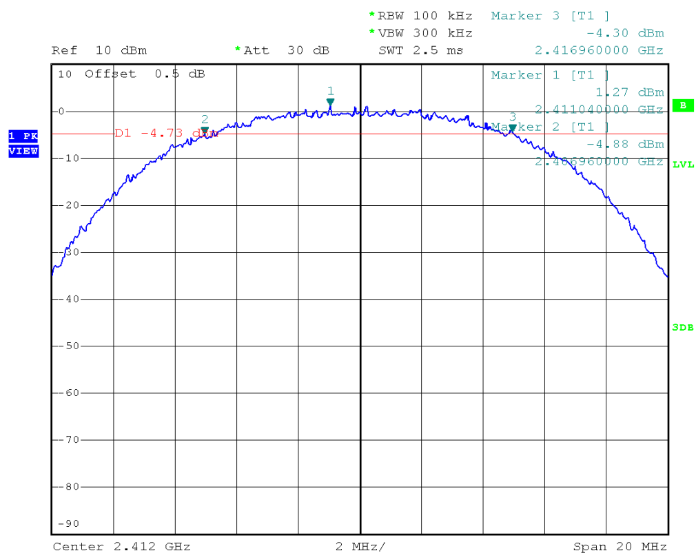
(Plot 2.2 A: Channel 1: 2412MHz @ 802.11b)
