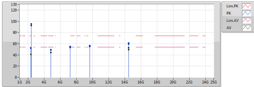
RE above 1GHz;Band:2.4G;11b;BWch:20MHz;Nss:1;Nant:1;Ch:2412MHz;TX
