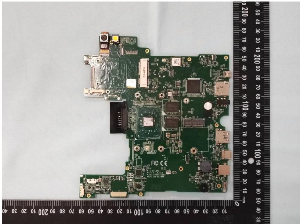
(24) EUT Photo
