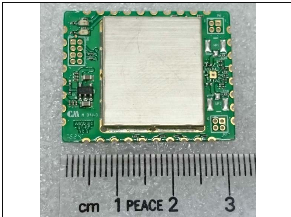
UHF Module
