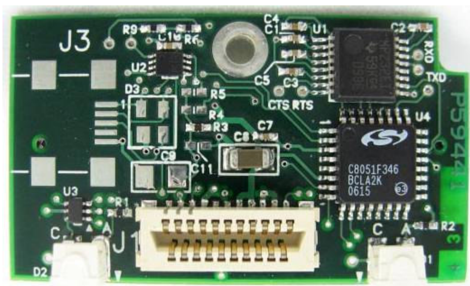
Controller PCA Side 1
