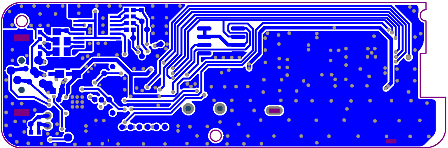
Bottom PCB
