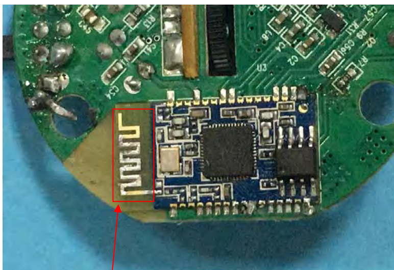
Antenna
