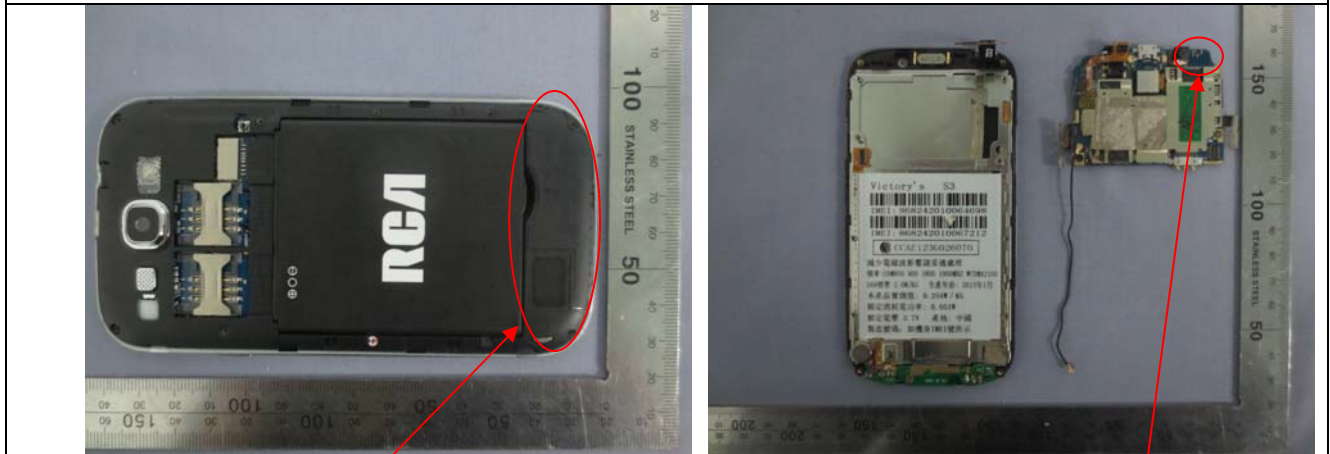
BT/WIFI ANT
