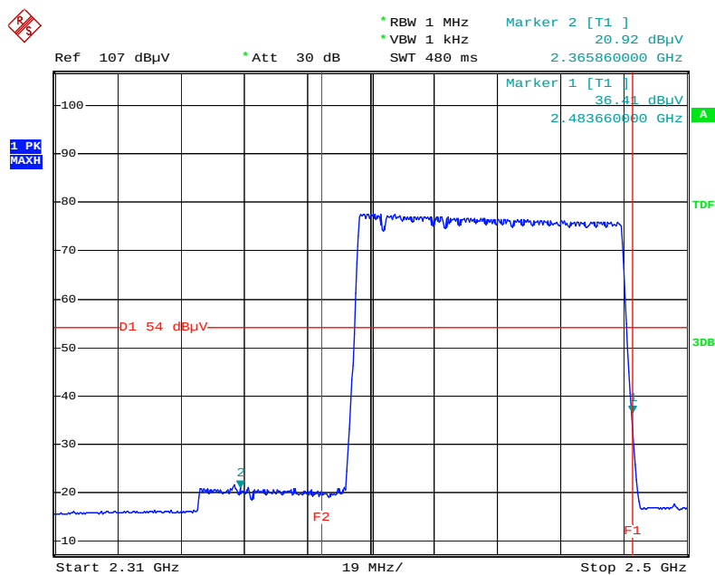
GFSK-hopping-Av
