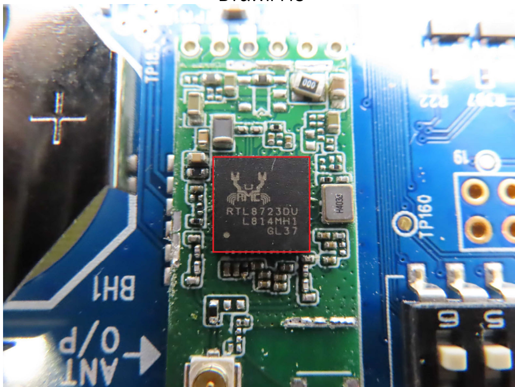
BT&amp;WIFI IC
