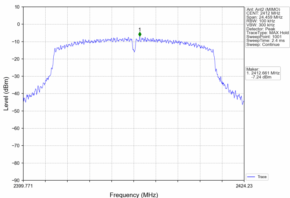
802.11n(HT20) LCH 2412MHz Ant2 (MIMO) NTV
