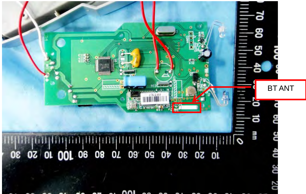
EUT Photo 3 )
