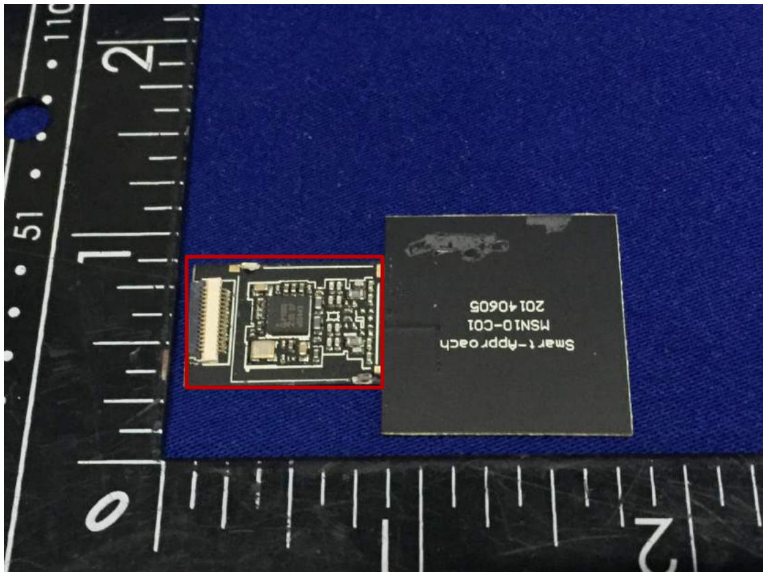
NFC Module
