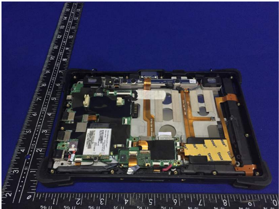
4G Module
