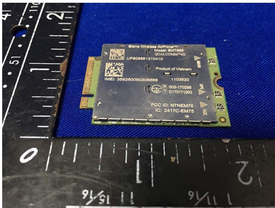
WCDMA/LTE module
