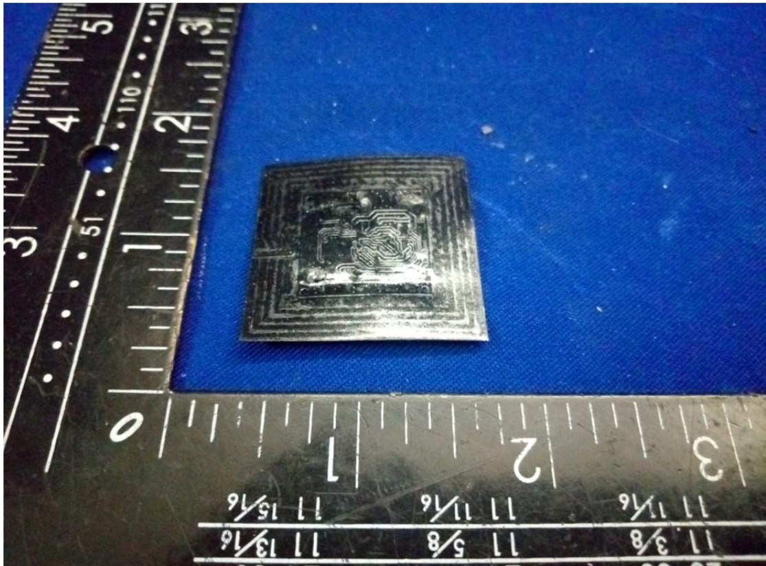
NFC Antenna
