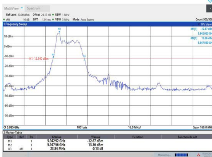
11AX80MIMO_Ant1_5985_52Tone_RU37
