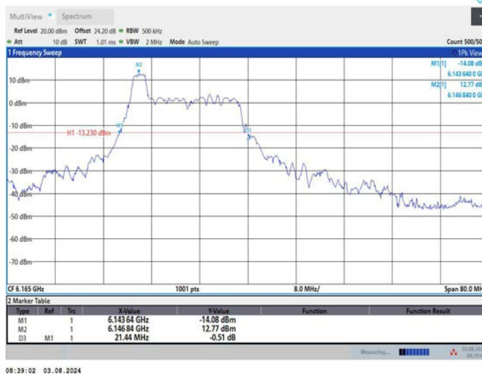
11AX40MIMO_Ant2_6165_52Tone_RU37
