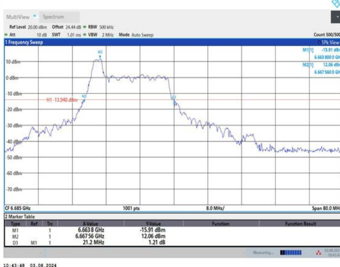
11AX40MIMO_Ant1_6685_52Tone_RU37
