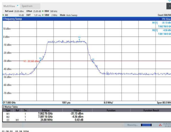
11AX40MIMO_Ant2_7085_26Tone_RU0
