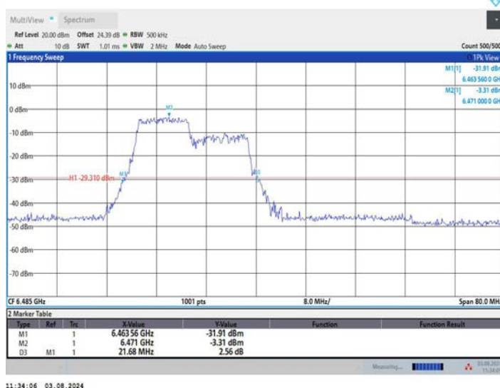
11AX40MIMO_Ant1_6485_242Tone_RU61
