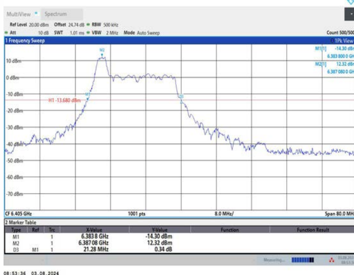
11AX40MIMO_Ant1_6405_52Tone_RU37
