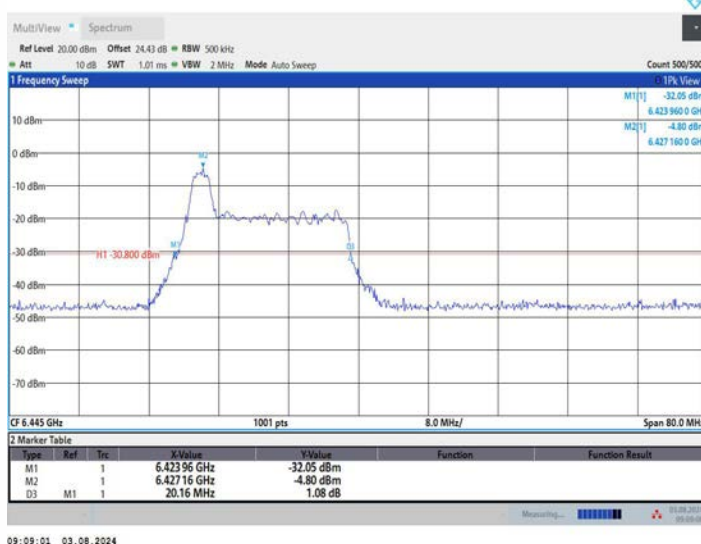
11AX40MIMO_Ant2_6445_52Tone_RU37
