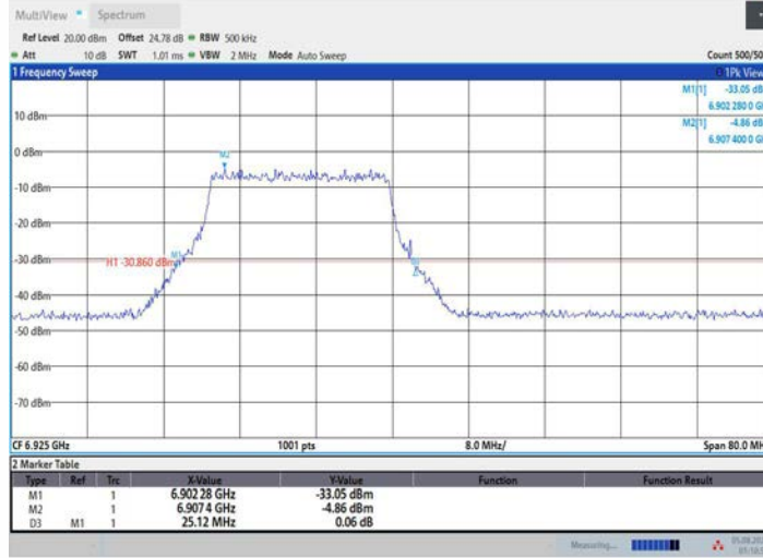
11AX40MIMO_Ant2_6925_26Tone_RU0
