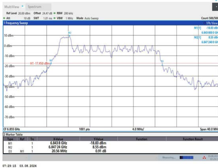
11AX20MIMO_Ant1_6855_52Tone_RU37
