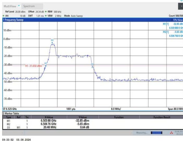
11AX40MIMO_Ant1_6525_52Tone_RU37
