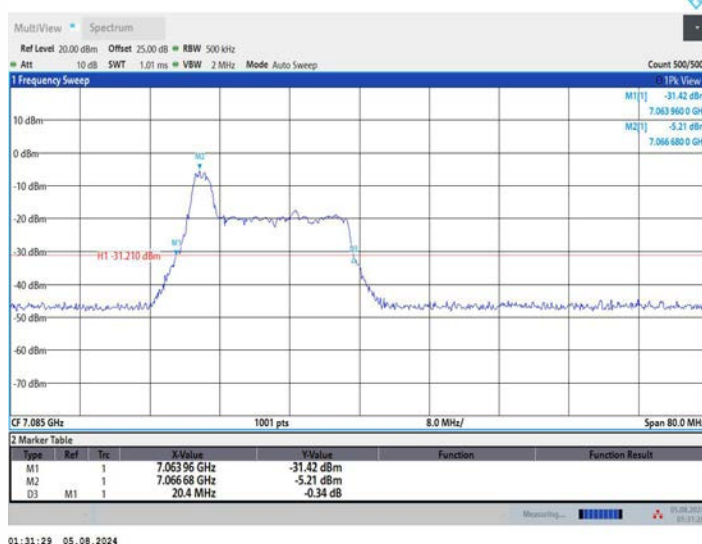
11AX40MIMO_Ant1_7085_52Tone_RU37
