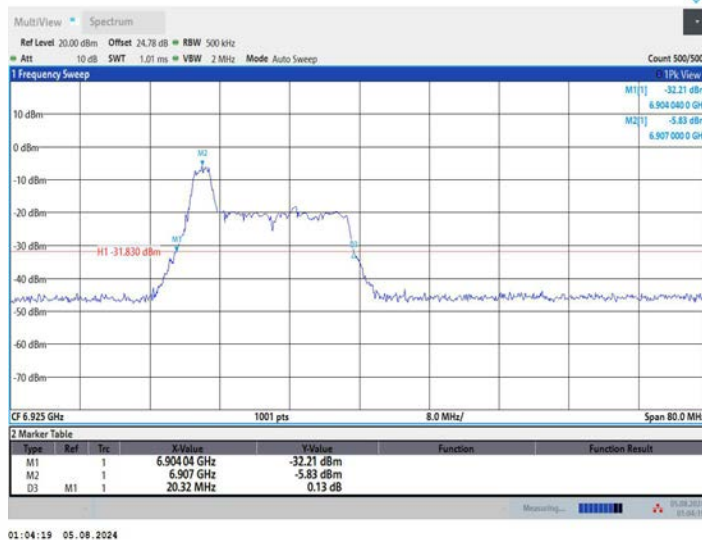
11AX40MIMO_Ant1_6925_52Tone_RU37
