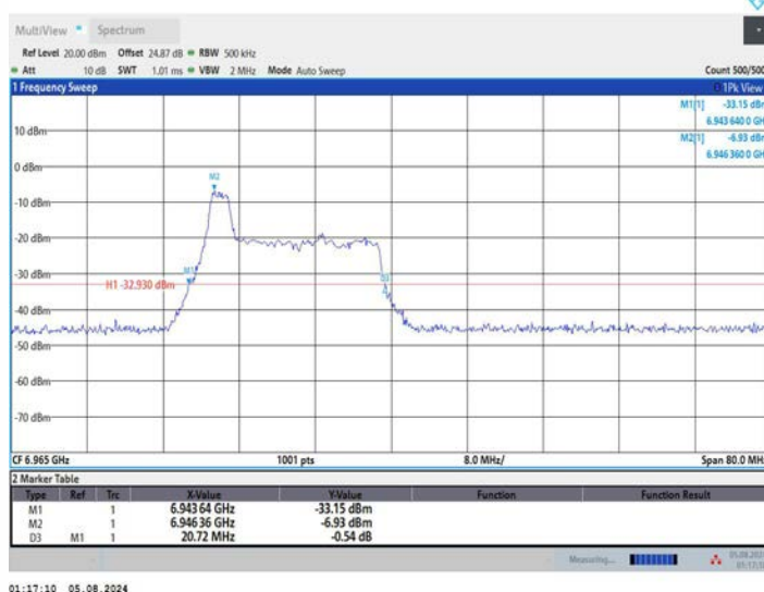
11AX40MIMO_Ant1_6965_52Tone_RU37
