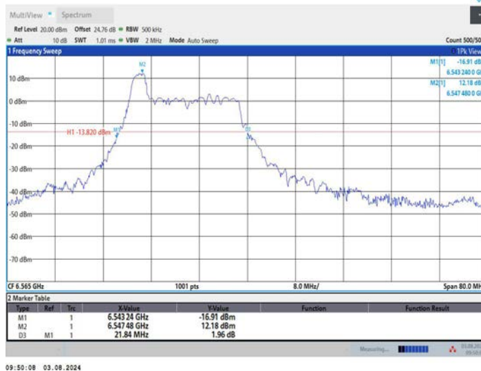
11AX40MIMO_Ant2_6565_52Tone_RU37
