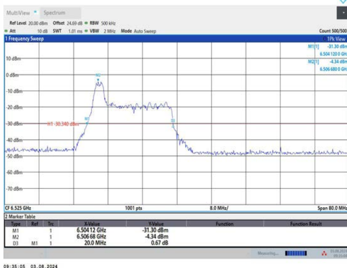
11AX40MIMO_Ant2_6525_52Tone_RU37
