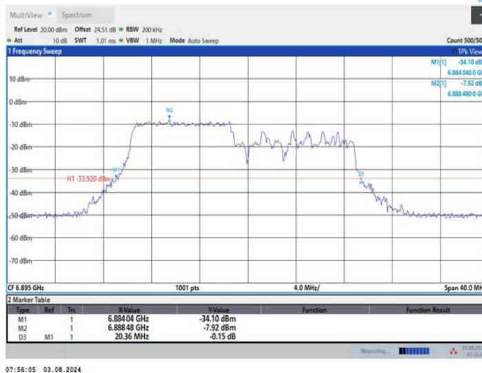
11AX20MIMO_Ant2_6895_26Tone_RU0
