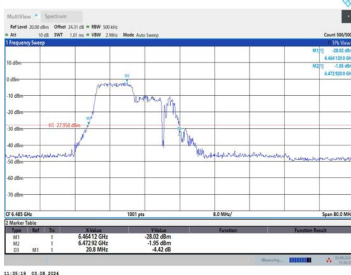
11AX40MIMO_Ant2_6485_242Tone_RU61
