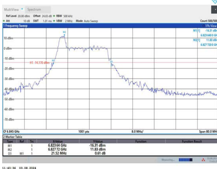
11AX40MIMO_Ant2_6845_52Tone_RU37
