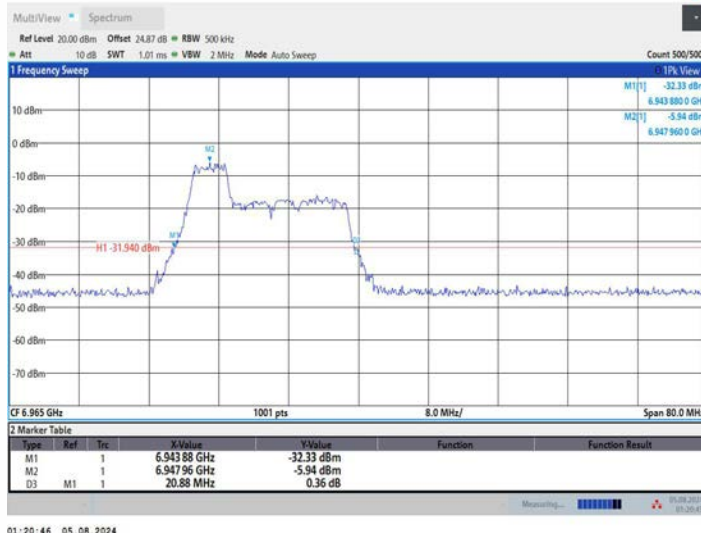
11AX40MIMO_Ant1_6965_106Tone_RU53
