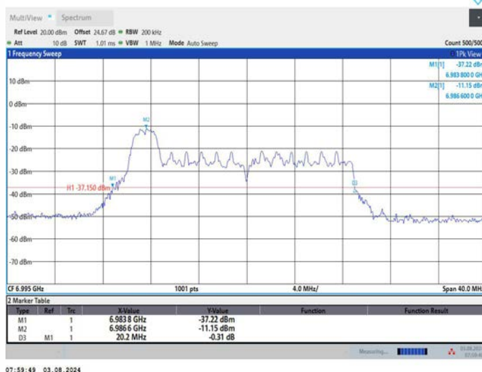
11AX20MIMO_Ant1_6995_52Tone_RU37
