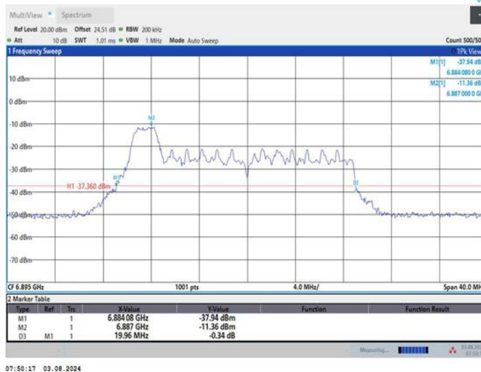
11AX20MIMO_Ant1_6895_52Tone_RU37
