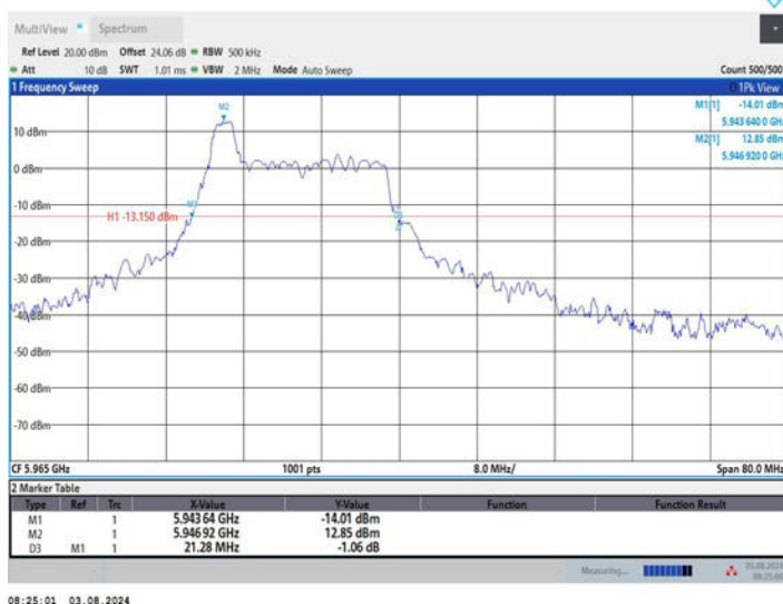
11AX40MIMO_Ant2_5965_52Tone_RU37
