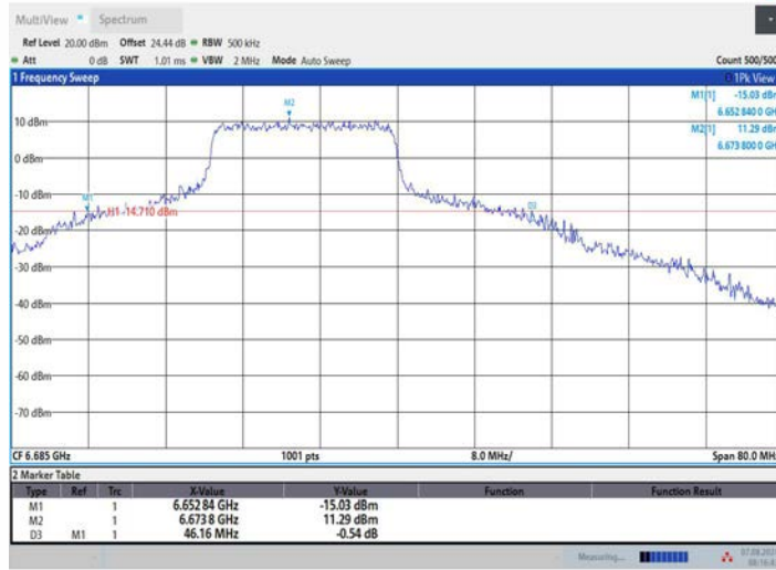
11AX40MIMO_Ant2_6685_26Tone_RU0
