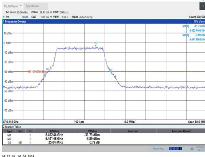
11AX40MIMO_Ant2_6445_26Tone_RU0
