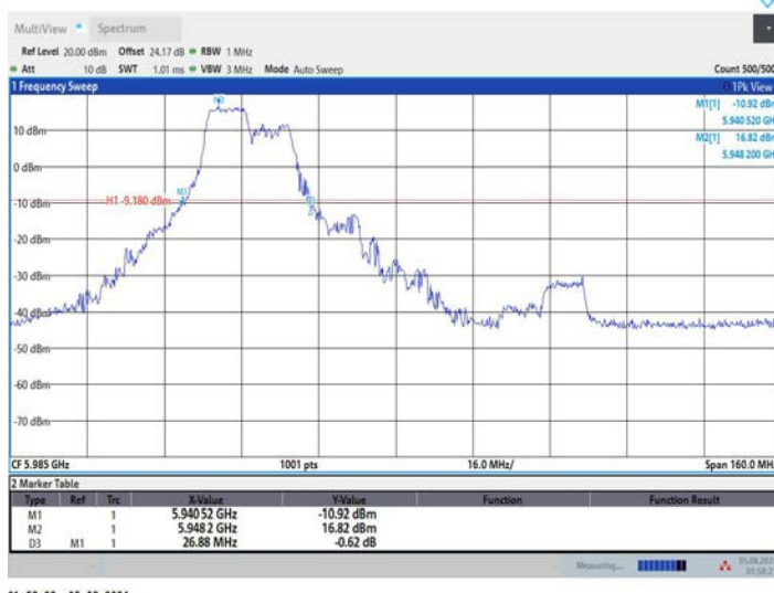
11AX80MIMO_Ant1_5985_242Tone_RU61
