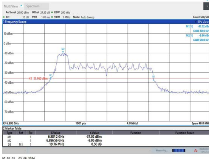
11AX20MIMO_Ant2_6895_52Tone_RU37
