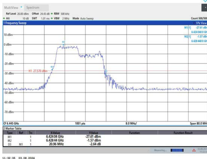
11AX40MIMO_Ant2_6445_242Tone_RU61
