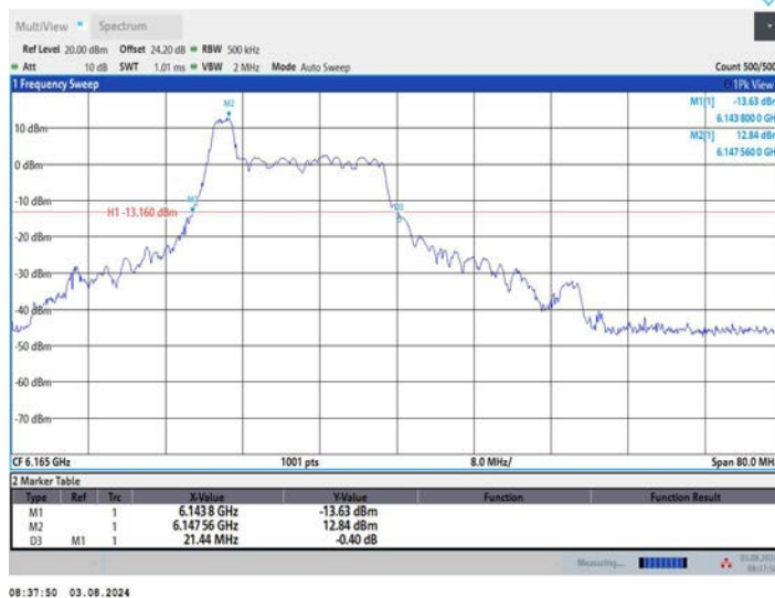
11AX40MIMO_Ant1_6165_52Tone_RU37
