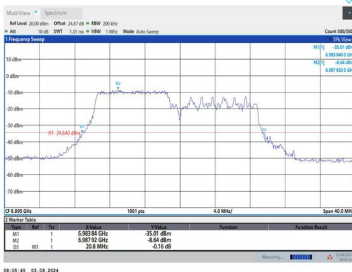
11AX20MIMO_Ant2_6995_26Tone_RU0
