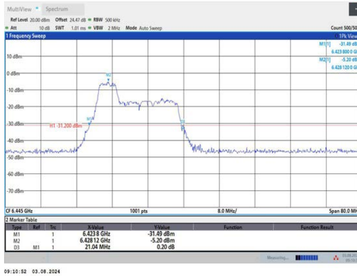
11AX40MIMO_Ant1_6445_106Tone_RU53
