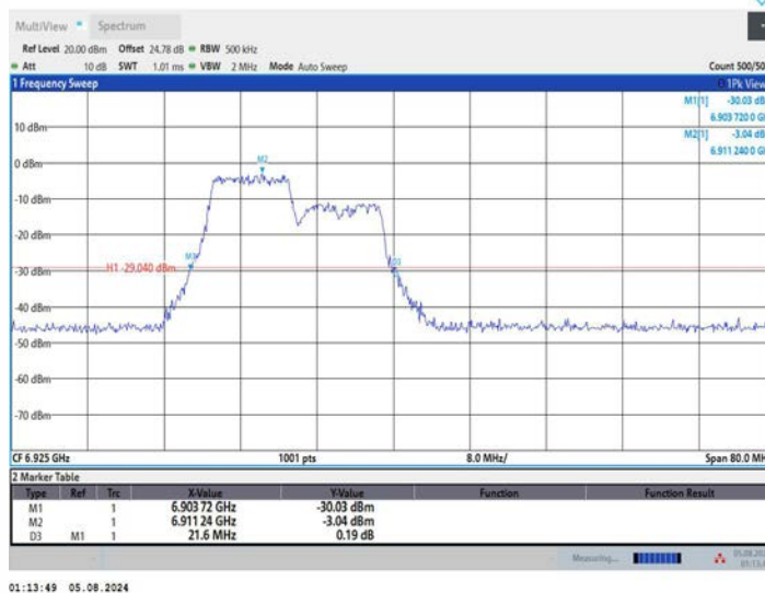
11AX40MIMO_Ant1_6925_242Tone_RU61
