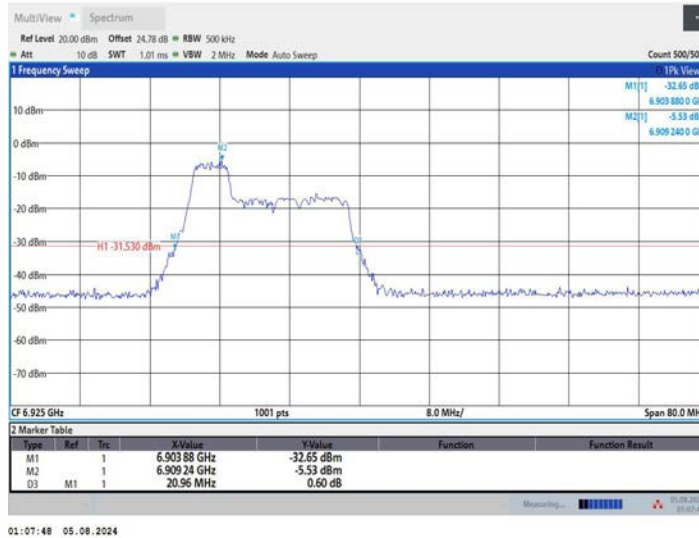
11AX40MIMO_Ant1_6925_106Tone_RU53
