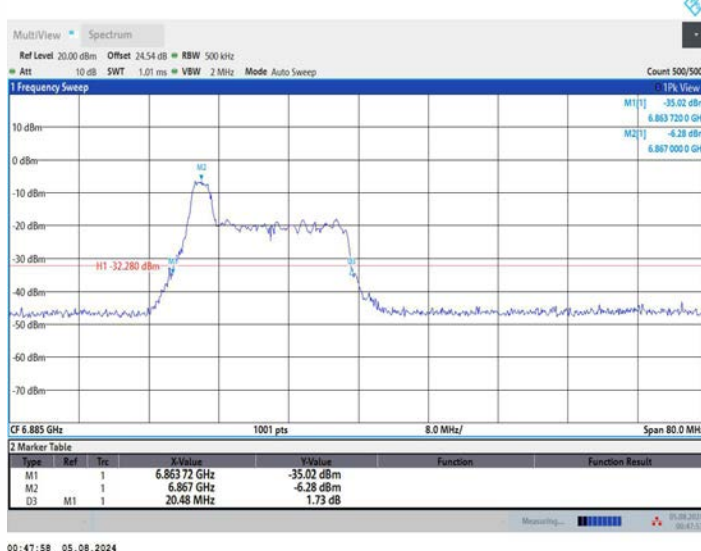
11AX40MIMO_Ant2_6885_52Tone_RU37
