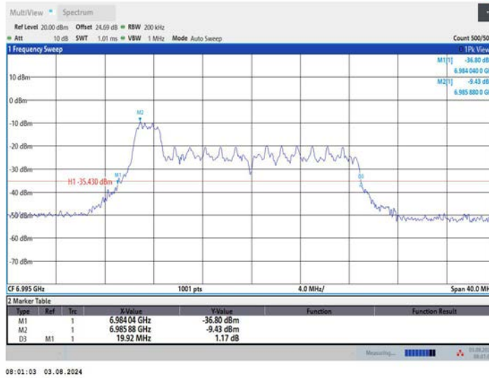
11AX20MIMO_Ant2_6995_52Tone_RU37
