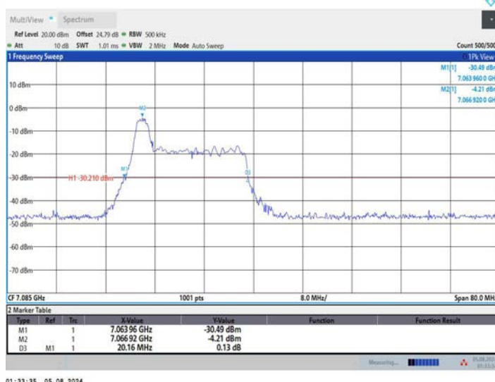
11AX40MIMO_Ant2_7085_52Tone_RU37
