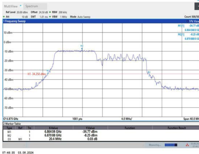
11AX20MIMO_Ant2_6875_26Tone_RU0
