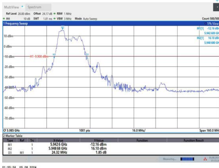
11AX80MIMO_Ant1_5985_106Tone_RU53
