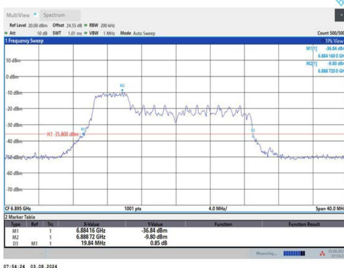
11AX20MIMO_Ant2_6895_106Tone_RU53
