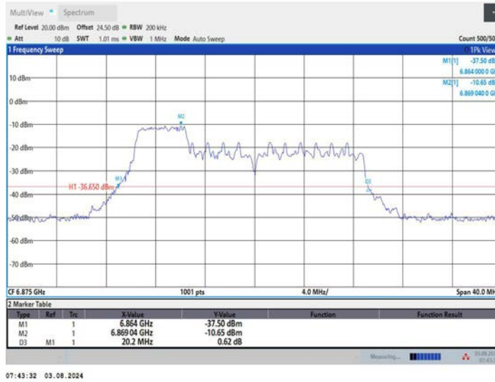
11AX20MIMO_Ant1_6875_106Tone_RU53
