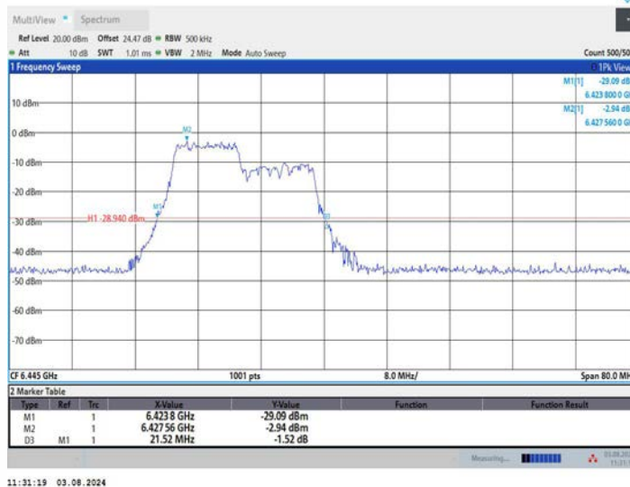
11AX40MIMO_Ant1_6445_242Tone_RU61
