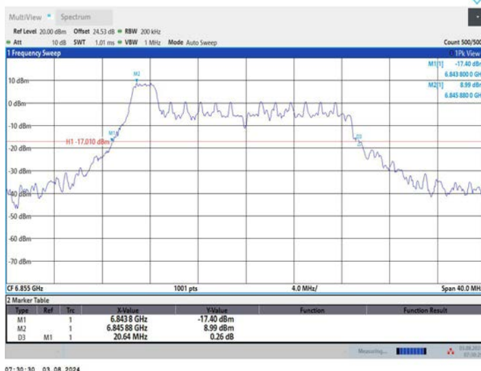
11AX20MIMO_Ant2_6855_52Tone_RU37
