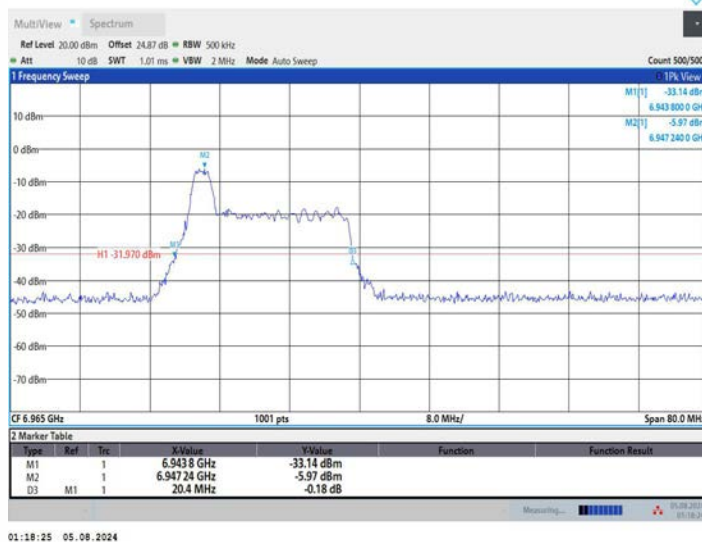
11AX40MIMO_Ant2_6965_52Tone_RU37
