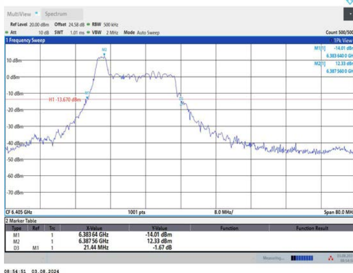
11AX40MIMO_Ant2_6405_52Tone_RU37
