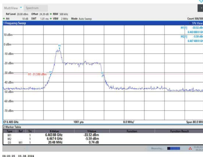
11AX40MIMO_Ant1_6485_52Tone_RU37
