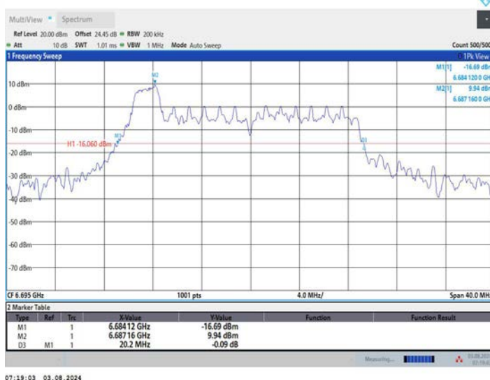
11AX20MIMO_Ant1_6695_52Tone_RU37
