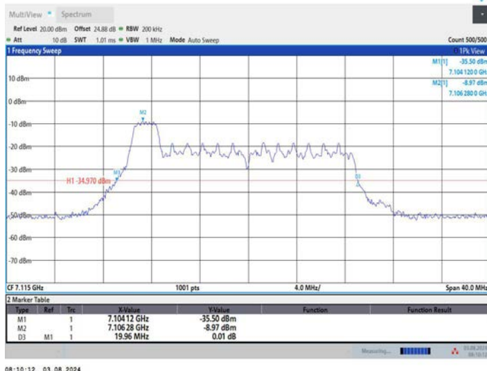
11AX20MIMO_Ant2_7115_52Tone_RU37
