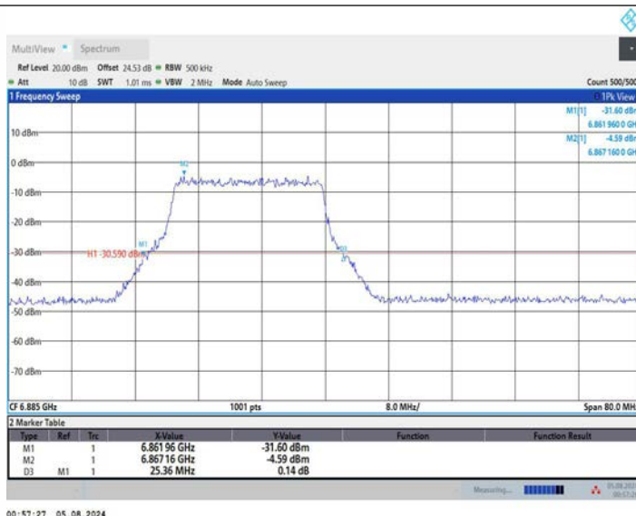
11AX40MIMO_Ant2_6885_26Tone_RU0
