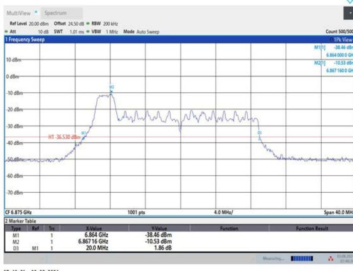
11AX20MIMO_Ant1_6875_52Tone_RU37
