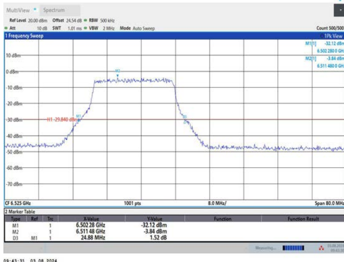
11AX40MIMO_Ant2_6525_26Tone_RU0
