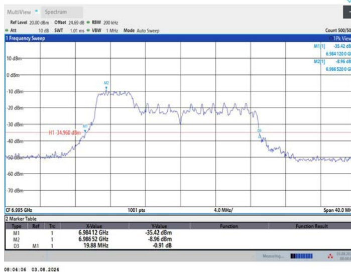
11AX20MIMO_Ant2_6995_106Tone_RU53
