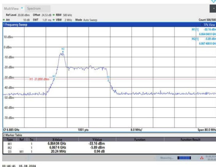
11AX40MIMO_Ant1_6885_52Tone_RU37
