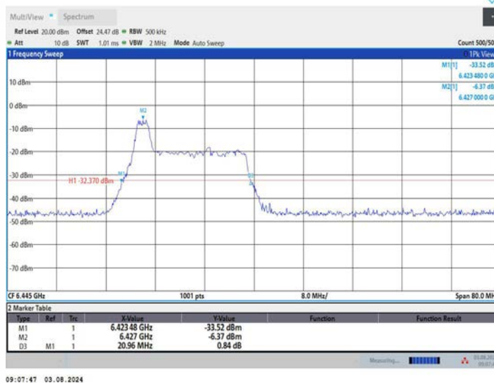
11AX40MIMO_Ant1_6445_52Tone_RU37
