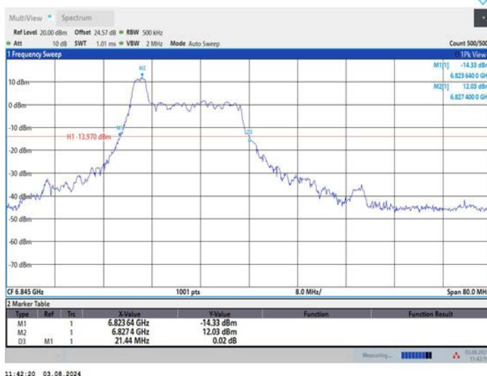
11AX40MIMO_Ant1_6845_52Tone_RU37
