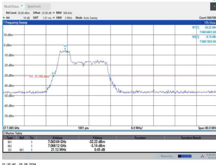
11AX40MIMO_Ant1_7085_106Tone_RU53
