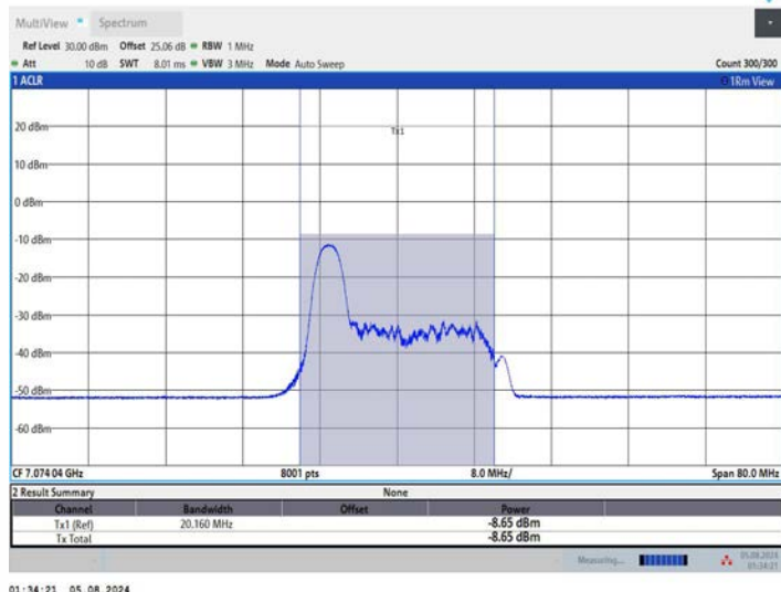
11AX40MIMO_Ant2_7085_52Tone_RU37
