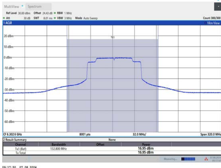
11AX160MIMO_Ant2_6345_996Tone_RU67
