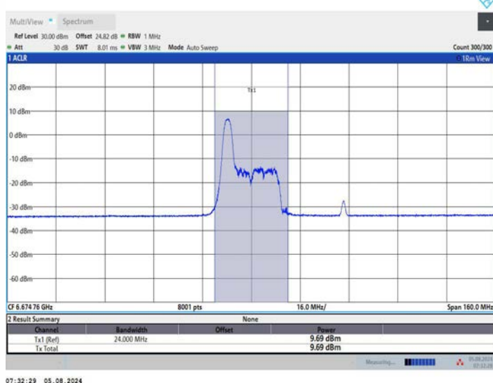
11AX80MIMO_Ant2_6705_52Tone_RU37
