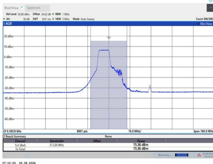
11AX80MIMO_Ant2_6625_242Tone_RU61
