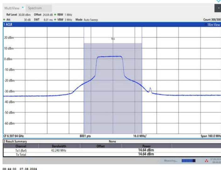
11AX80MIMO_Ant1_6625_484Tone_RU65
