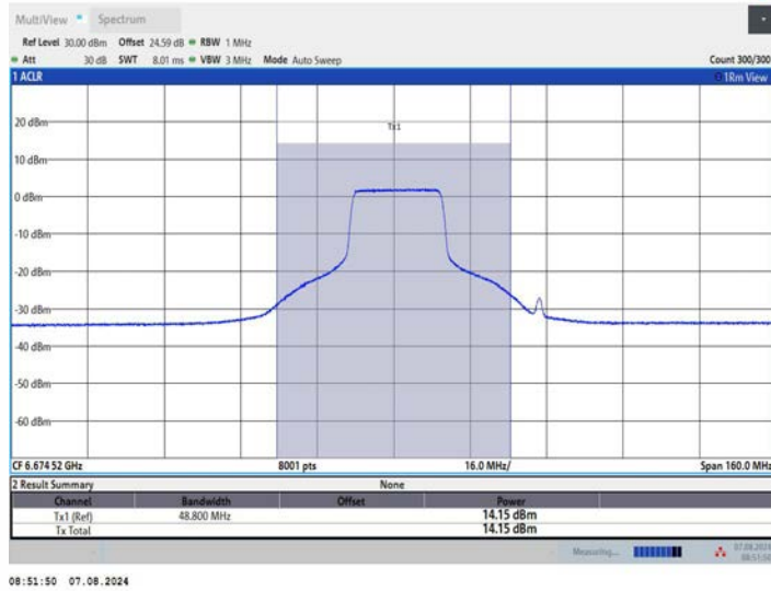
11AX80MIMO_Ant2_6705_484Tone_RU65
