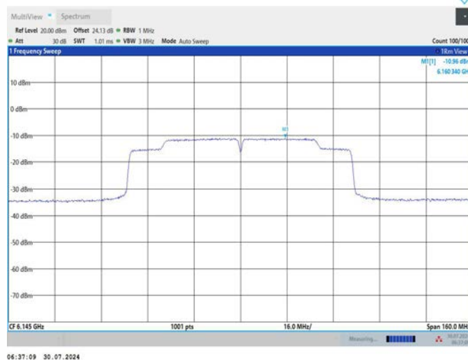
11AC80MIMO_Ant2_6145
