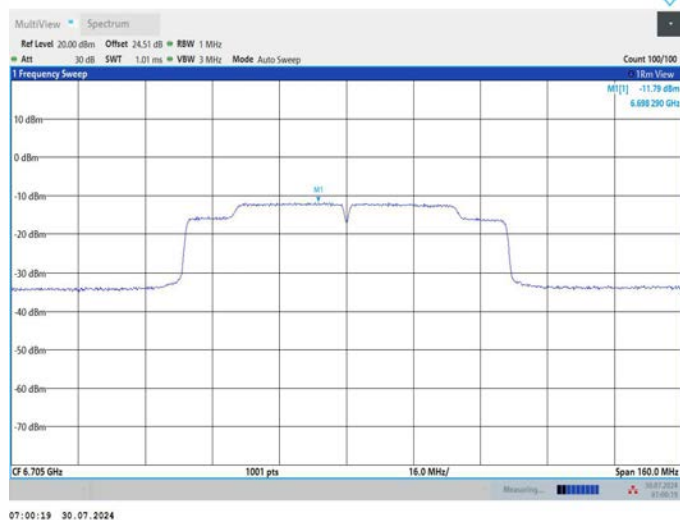
11AC80MIMO_Ant1_6705
