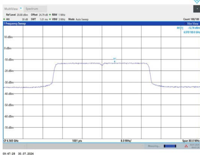
11AX40MIMO_Ant2_6565
