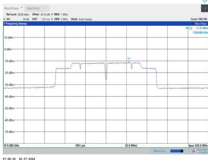
11AC160MIMO_Ant2_6985
