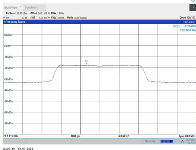
11AC20MIMO_Ant2_7115
