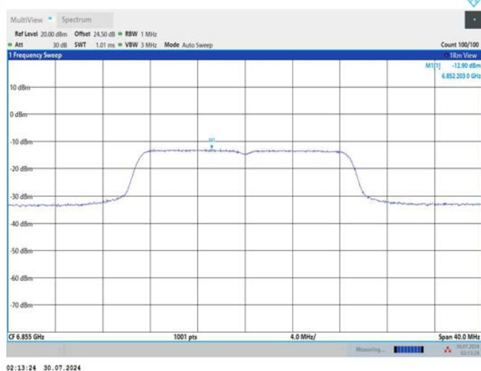
11AC20MIMO_Ant1_6855
