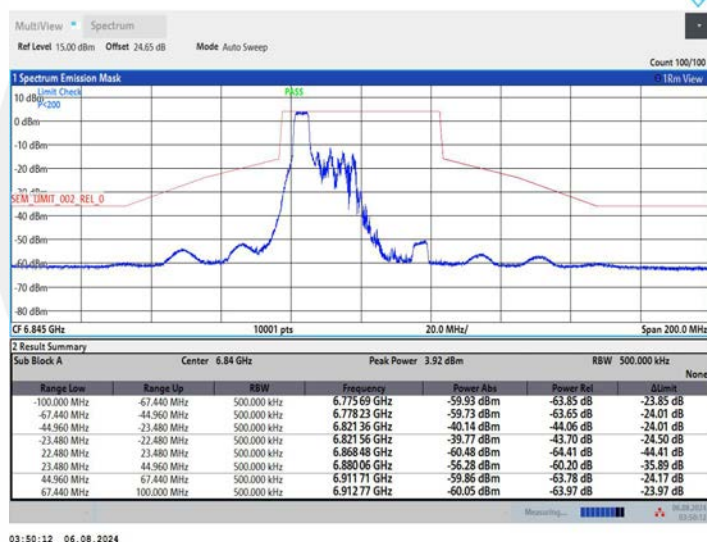
11AX40MIMO_Ant2_6845_106Tone_RU53
