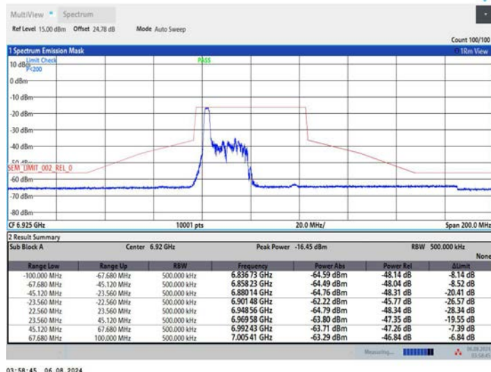
11AX40MIMO_Ant1_6925_52Tone_RU37
