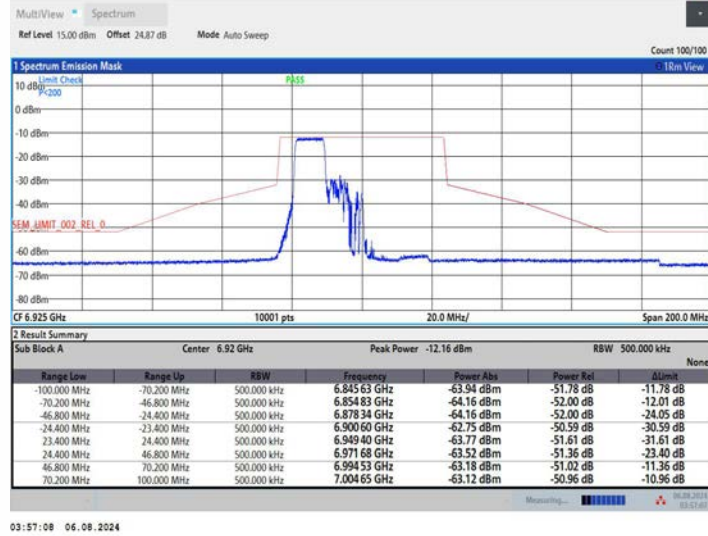
11AX40MIMO_Ant2_6925_242Tone_RU61
