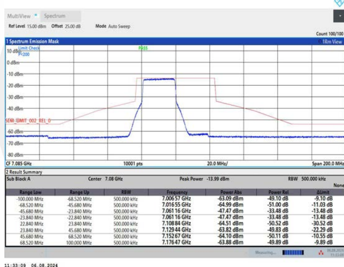
11AX40MIMO_Ant2_7085_26Tone_RU0
