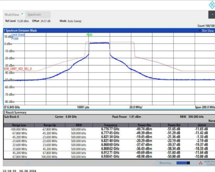
11AX40MIMO_Ant2_6845_26Tone_RU0
