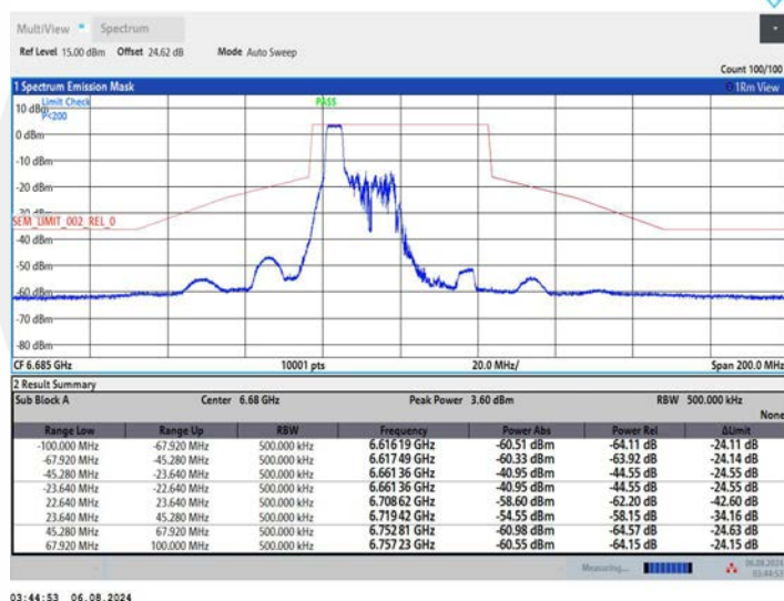
11AX40MIMO_Ant2_6685_106Tone_RU53
