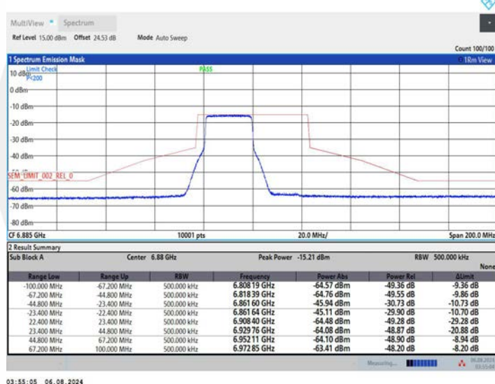
11AX40MIMO_Ant2_6885_26Tone_RU0
