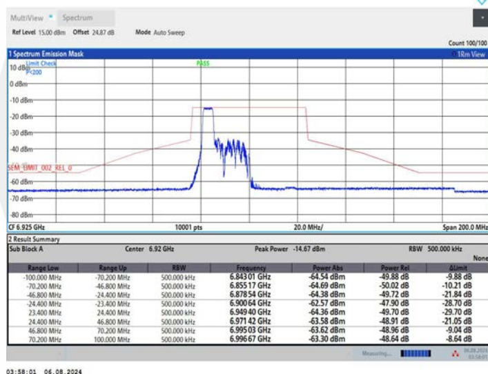
11AX40MIMO_Ant2_6925_106Tone_RU53
