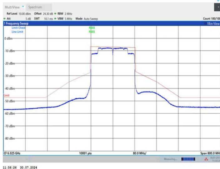
11AX160MIMO_Ant2_6025
