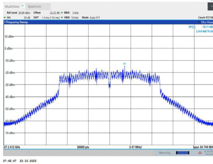
11G_Ant2_2412
