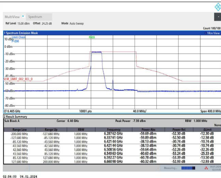
11AX80MIMO_Ant1_6465_484Tone_RU65
