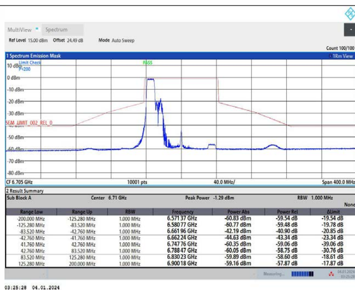
11AX80MIMO_Ant2_6705_242Tone_RU61
