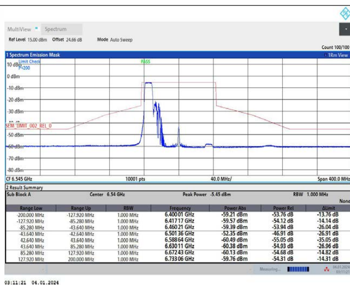
11AX80MIMO_Ant2_6545_242Tone_RU61
