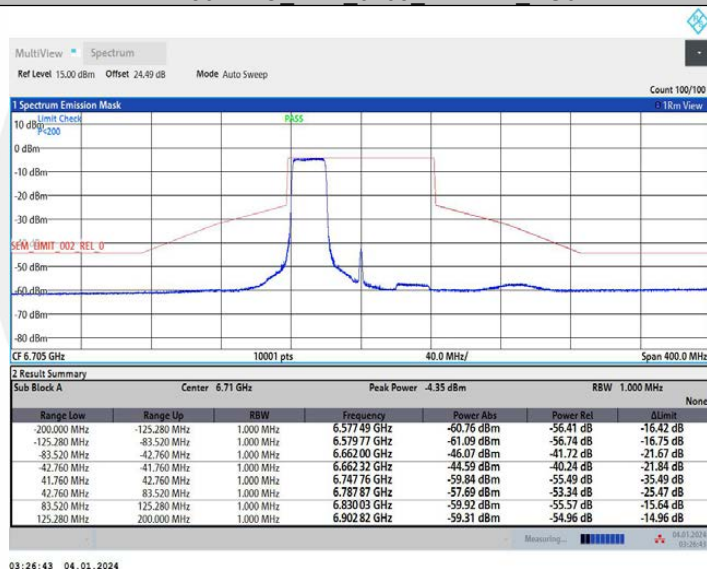
11AX80MIMO_Ant2_6705_484Tone_RU65
