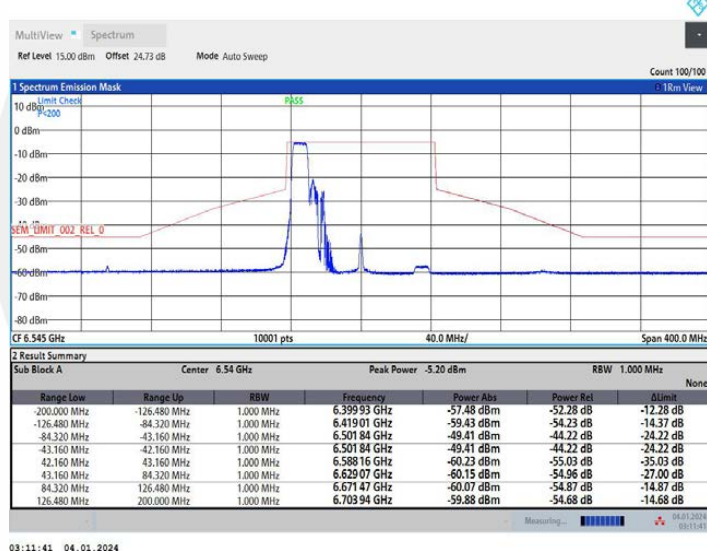
11AX80MIMO_Ant1_6545_242Tone_RU61
