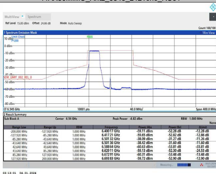
11AX80MIMO_Ant2_6545_484Tone_RU65
