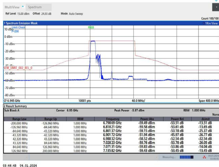
11AX80MIMO_Ant2_6945_242Tone_RU61
