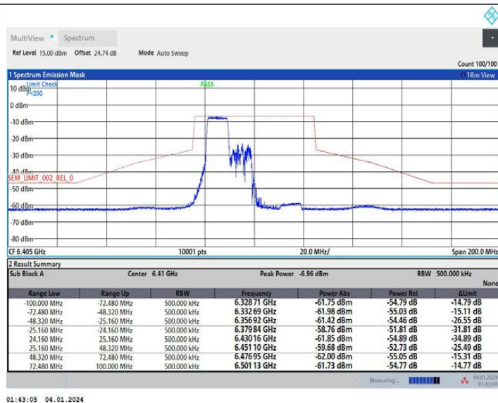
11AX40MIMO_Ant2_6405_242Tone_RU61
