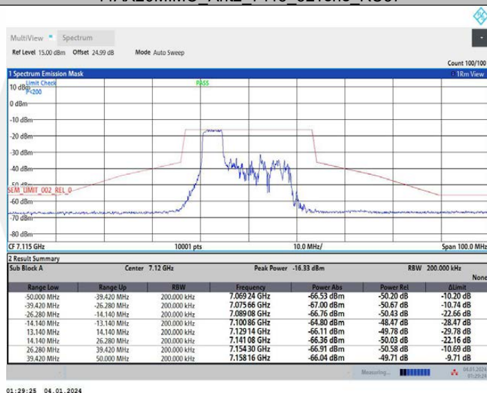
11AX20MIMO_Ant2_7115_106Tone_RU53
