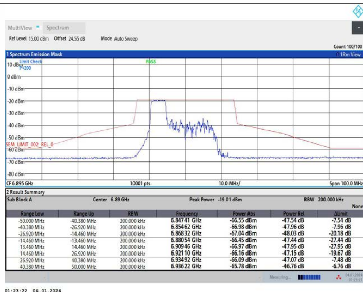
11AX20MIMO_Ant1_6895_106Tone_RU53
