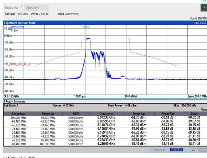
11AX40MIMO_Ant1_6165_106Tone_RU53
