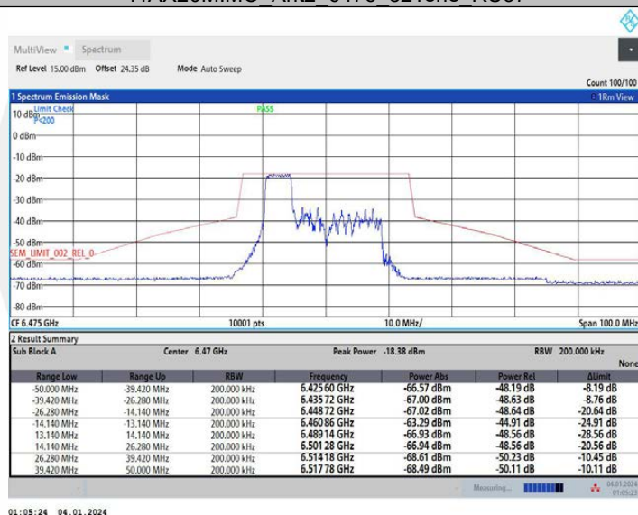
11AX20MIMO_Ant2_6475_106Tone_RU53
