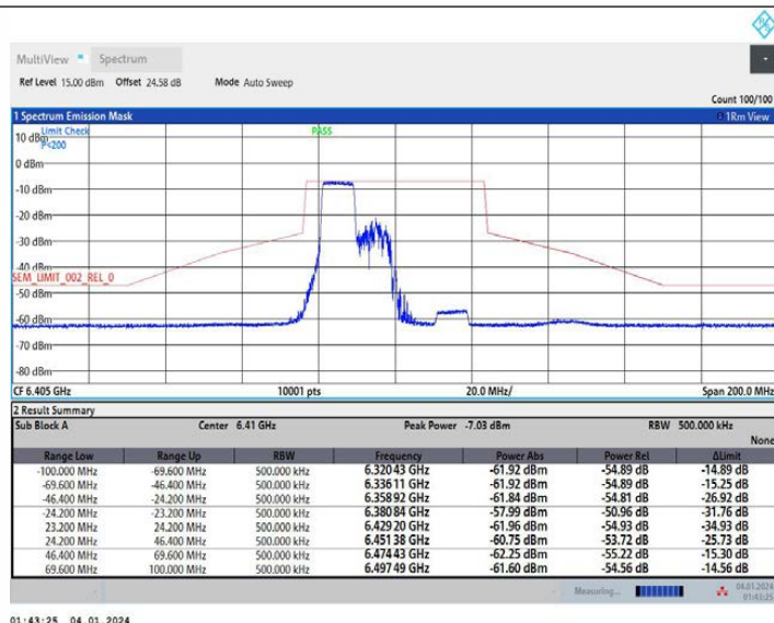
11AX40MIMO_Ant1_6405_242Tone_RU61
