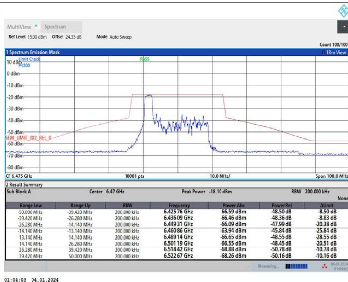
11AX20MIMO_Ant2_6475_52Tone_RU37
