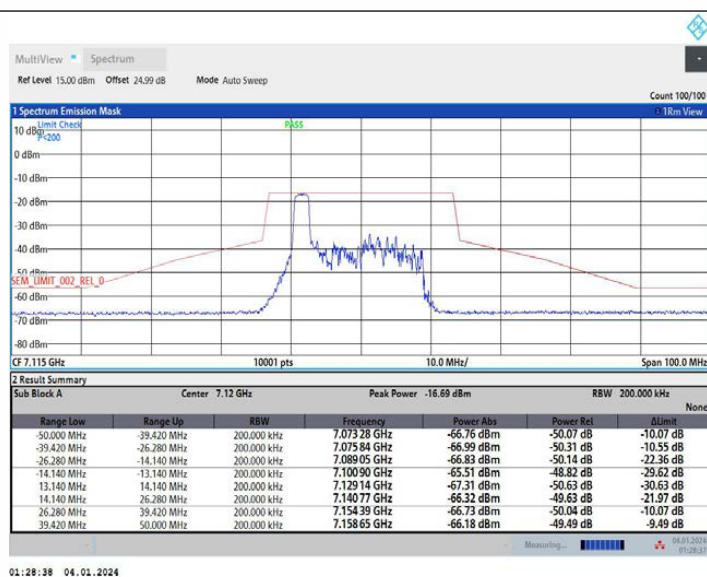
11AX20MIMO_Ant2_7115_52Tone_RU37
