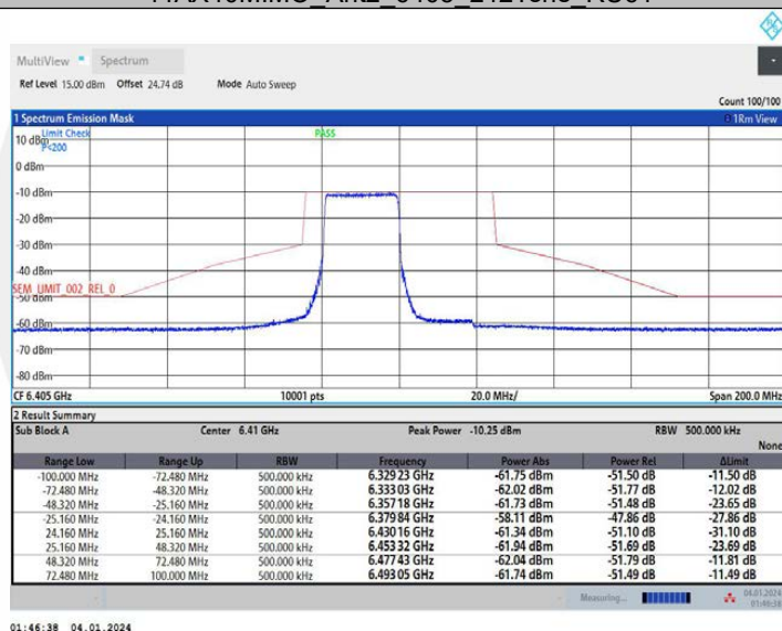
11AX40MIMO_Ant1_6405_26Tone_RU0
