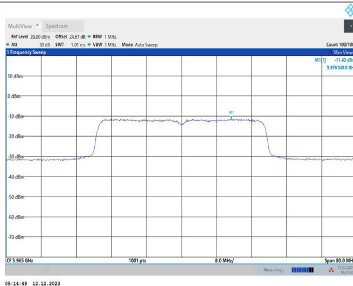
11AX40MIMO_Ant1_5965
