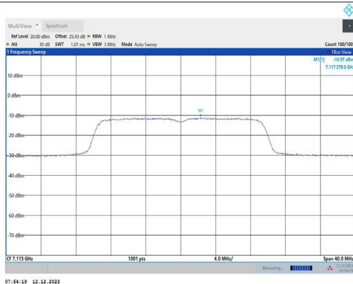
11AX20MIMO_Ant1_7115
