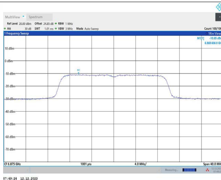
11AX20MIMO_Ant1_6875
