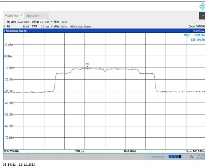
11AX80MIMO_Ant1_6705
