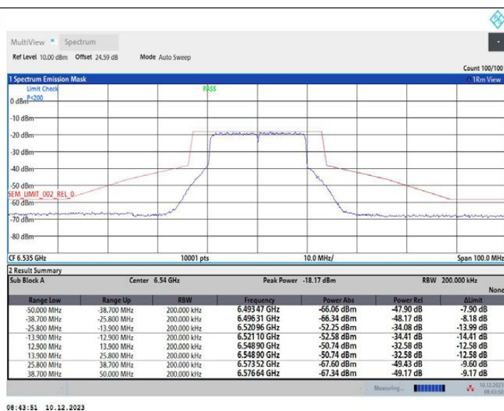
11AX20MIMO_Ant1_6535
