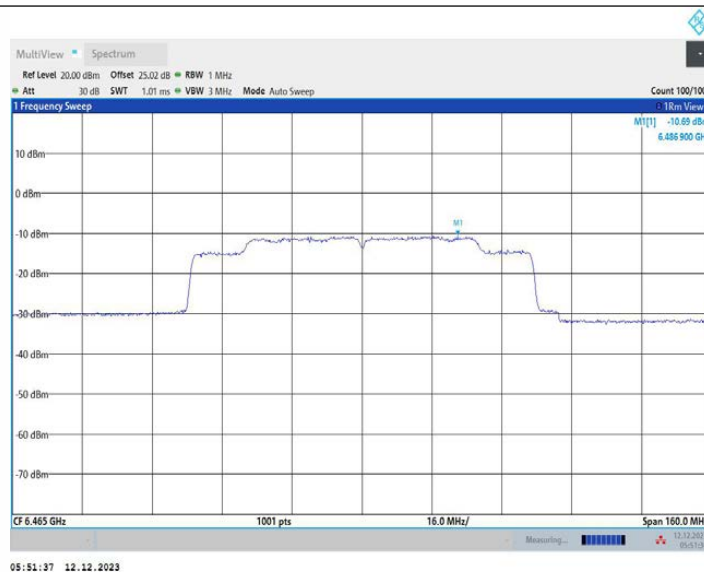
11AX80MIMO_Ant1_6465
