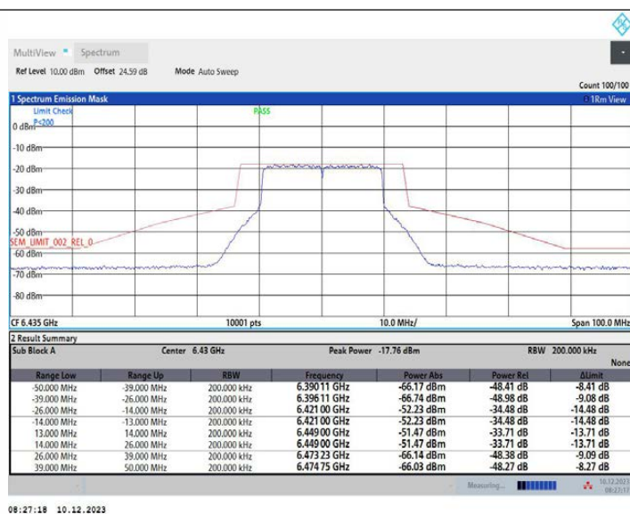
11AX20MIMO_Ant1_6435
