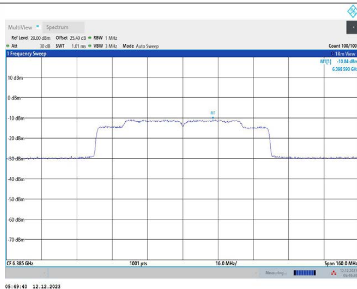
11AX80MIMO_Ant1_6385
