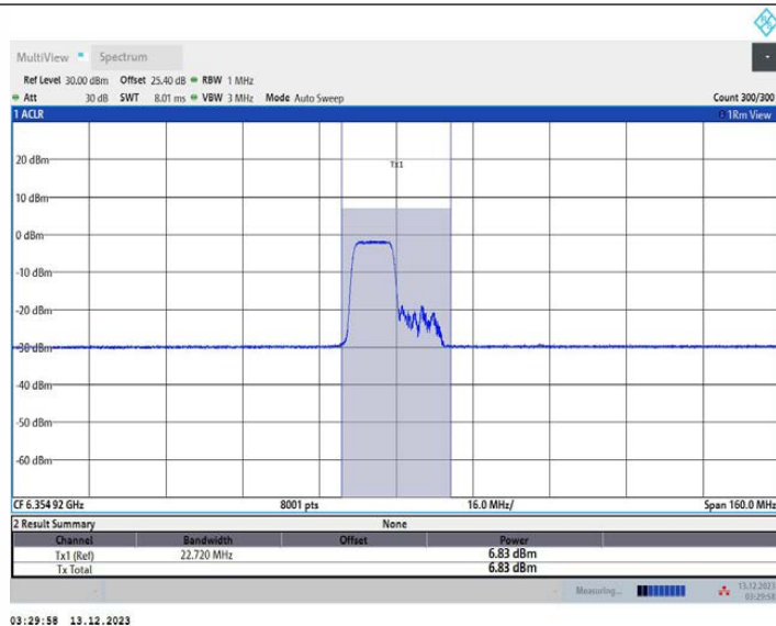
11AX80MIMO_Ant2_6385_242Tone_RU61
