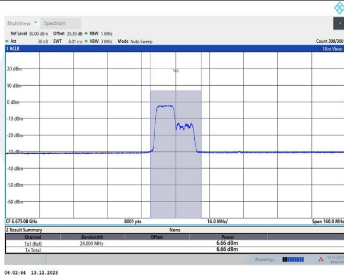
11AX80MIMO_Ant1_6705_242Tone_RU61
