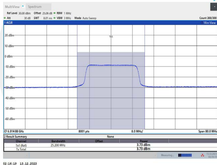
11AX40MIMO_Ant1_6925_26Tone_RU0
