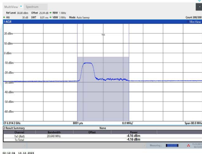
11AX40MIMO_Ant1_6925_106Tone_RU53
