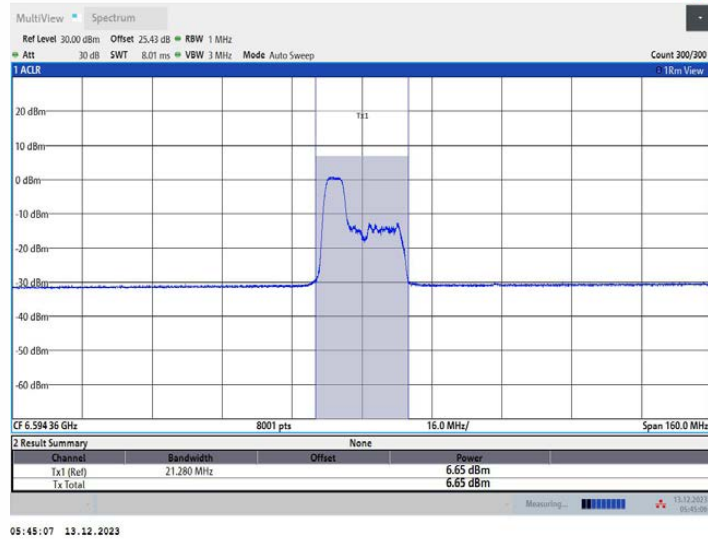
11AX80MIMO_Ant1_6625_106Tone_RU53
