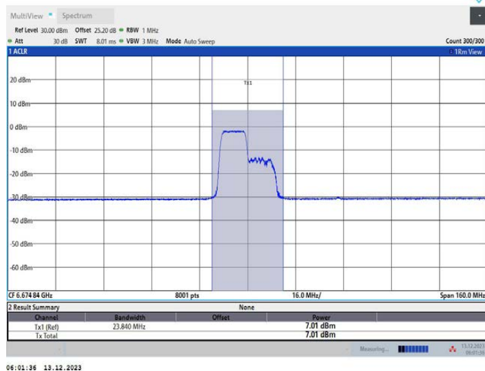
11AX80MIMO_Ant2_6705_242Tone_RU61
