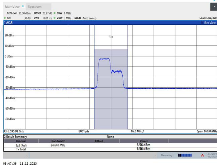
11AX80MIMO_Ant1_6625_242Tone_RU61
