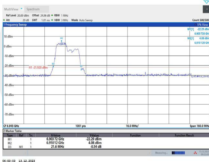
11AX80MIMO_Ant1_6945_242Tone_RU61
