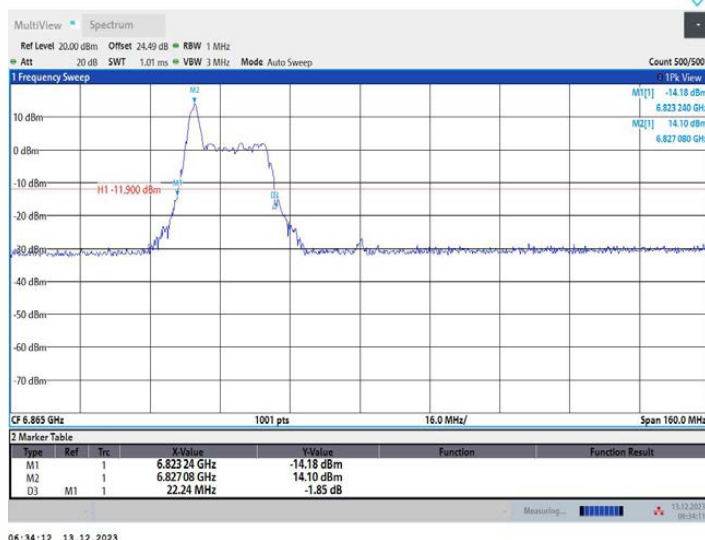
11AX80MIMO_Ant2_6865_52Tone_RU37
