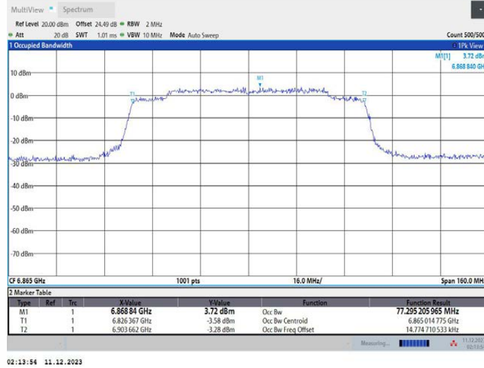
11AX80MIMO_Ant1_6865
