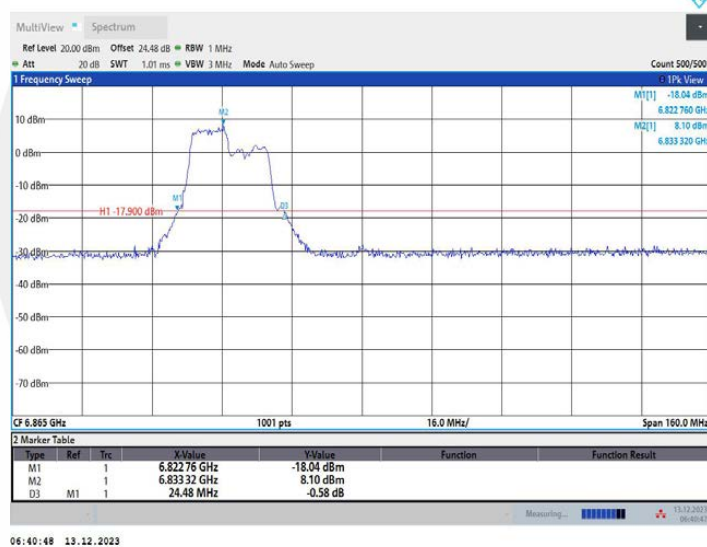
11AX80MIMO_Ant1_6865_242Tone_RU61
