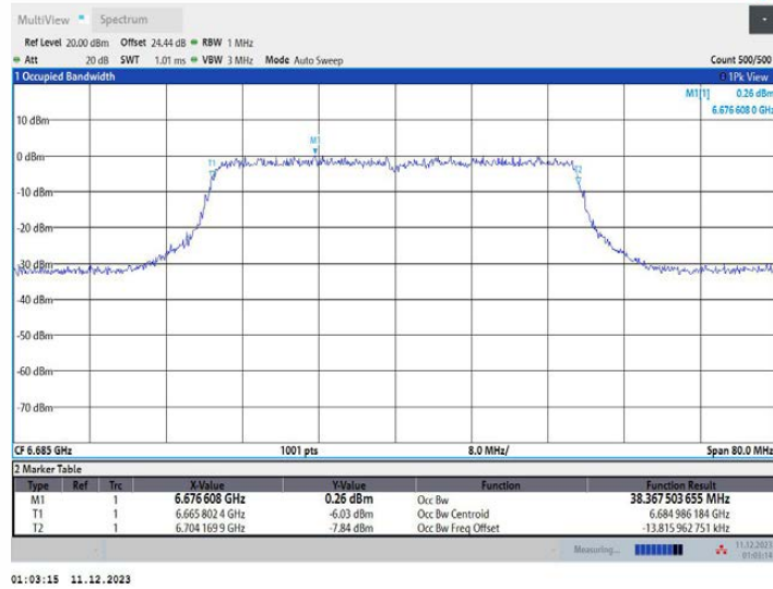
11AX40MIMO_Ant1_685
