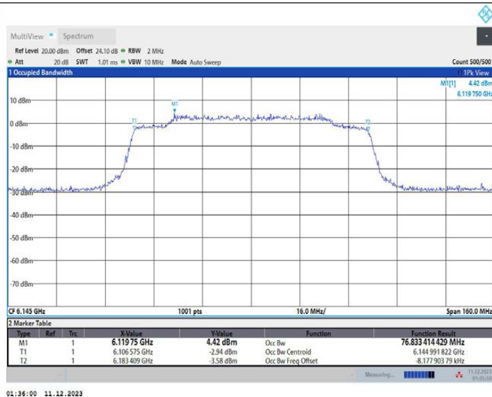
11AX80MIMO_Ant1_6145
