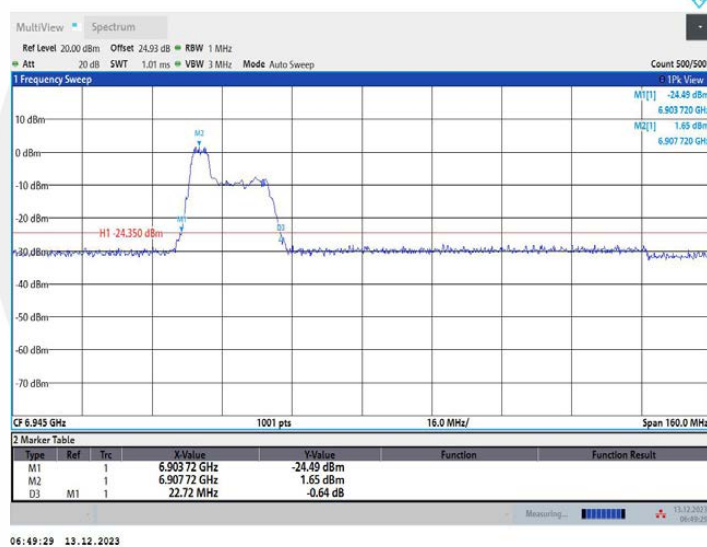
11AX80MIMO_Ant2_6945_106Tone_RU53
