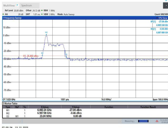
11AX80MIMO_Ant2_7025_52Tone_RU37
