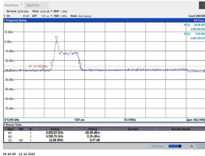
11AX80MIMO_Ant2_6945_52Tone_RU37
