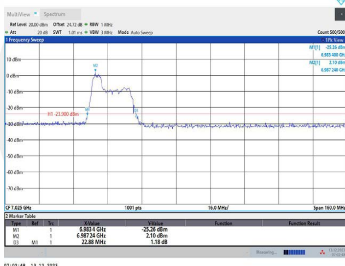
11AX80MIMO_Ant2_7025_106Tone_RU53
