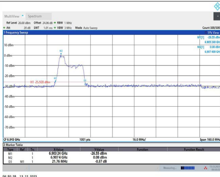
11AX80MIMO_Ant1_6945_106Tone_RU53
