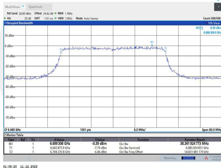
11AX40MIMO_Ant2_685
