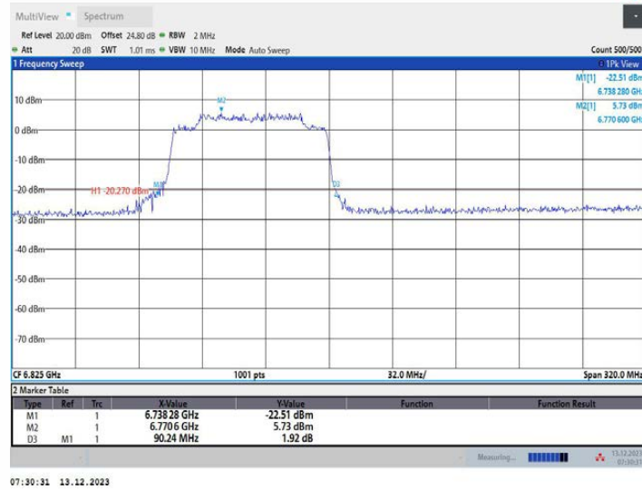
11AX160MIMO_Ant1_6825_996Tone_RU67
