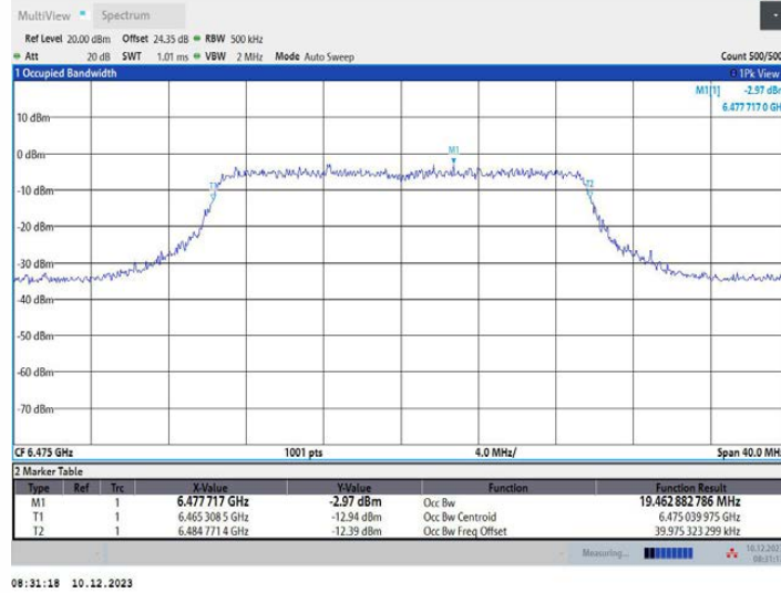
11AX20MIMO_Ant1_6475
