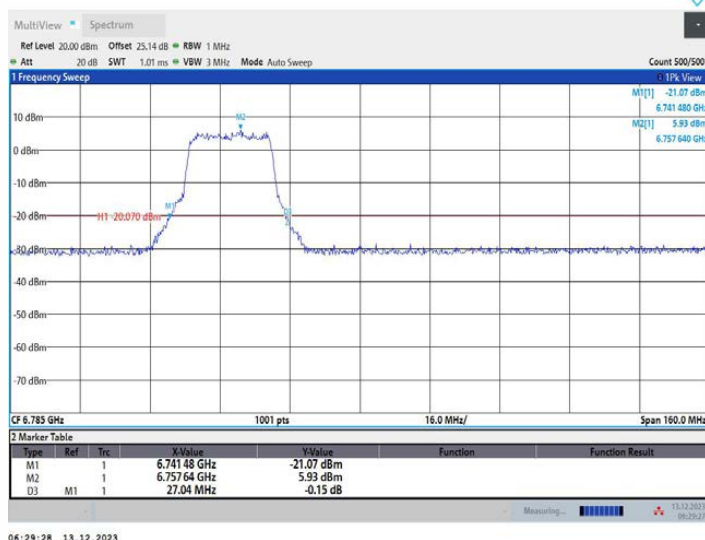
11AX80MIMO_Ant1_6785_484Tone_RU65
