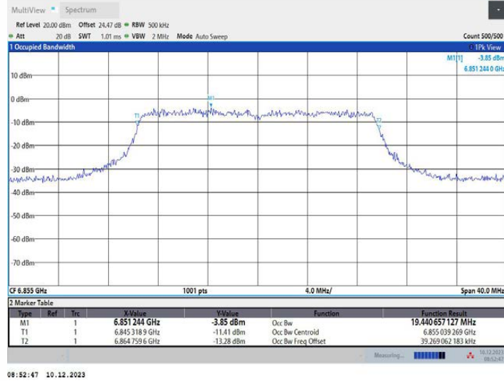
11AX20MIMO_Ant1_6855
