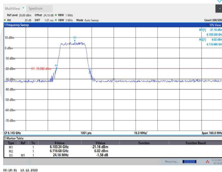
11AX80MIMO_Ant2_6145_484Tone_RU65
