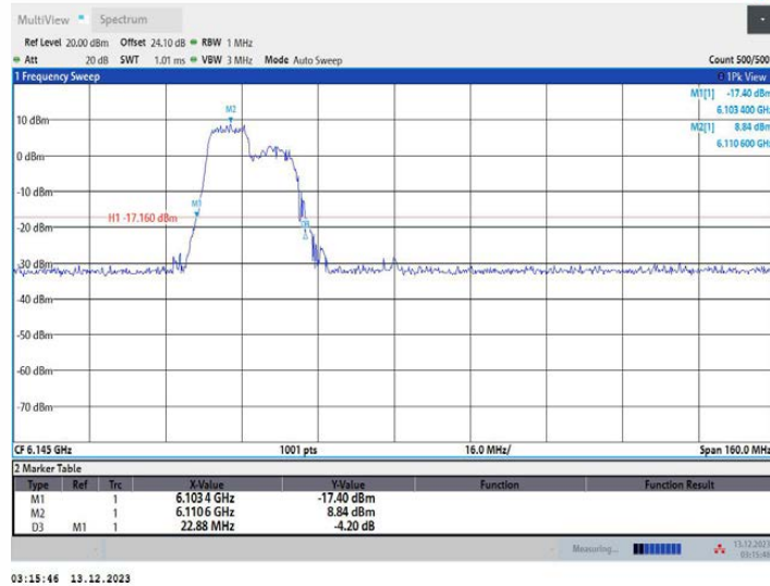
11AX80MIMO_Ant2_6145_242Tone_RU61
