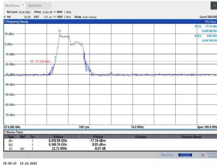
11AX80MIMO_Ant2_6385_242Tone_RU61
