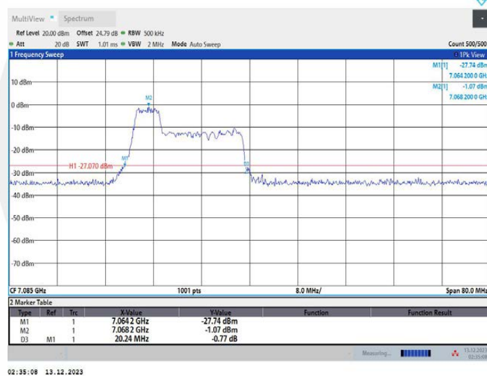
11AX40MIMO_Ant1_7085_106Tone_RU53
