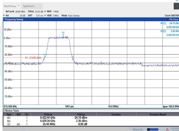
11AX80MIMO_Ant2_6465_484Tone_RU65
