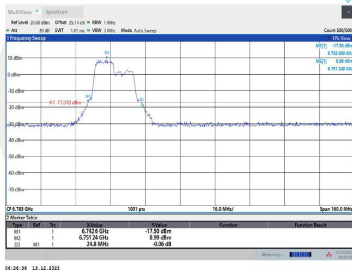
11AX80MIMO_Ant1_6785_242Tone_RU61
