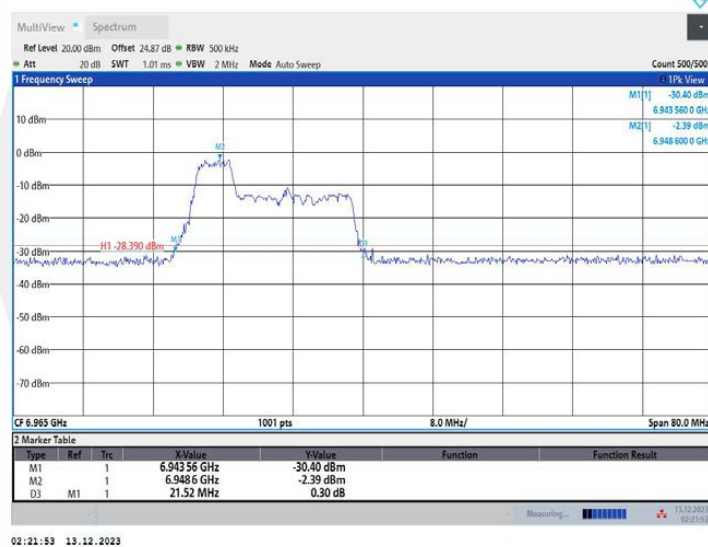
11AX40MIMO_Ant2_6965_106Tone_RU53
