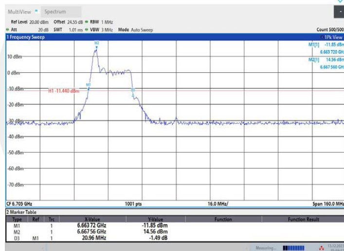
11AX80MIMO_Ant1_6705_52Tone_RU37
