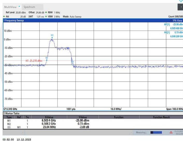
11AX80MIMO_Ant2_6545_106Tone_RU53
