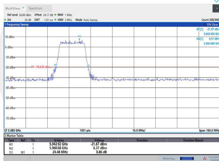
11AX80MIMO_Ant2_5985_484Tone_RU65
