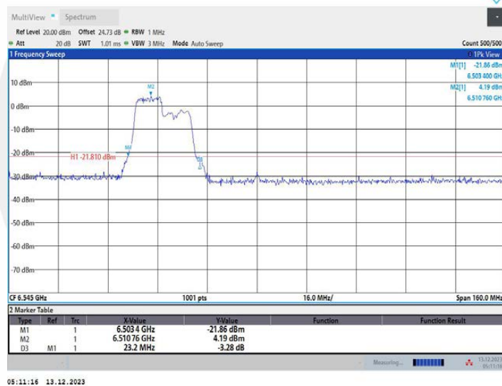
11AX80MIMO_Ant1_6545_242Tone_RU61
