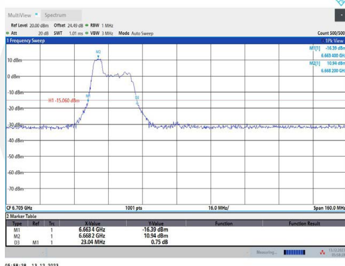
11AX80MIMO_Ant2_6705_106Tone_RU53
