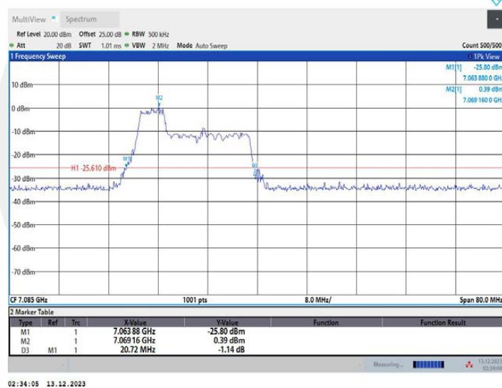
11AX40MIMO_Ant2_7085_106Tone_RU53
