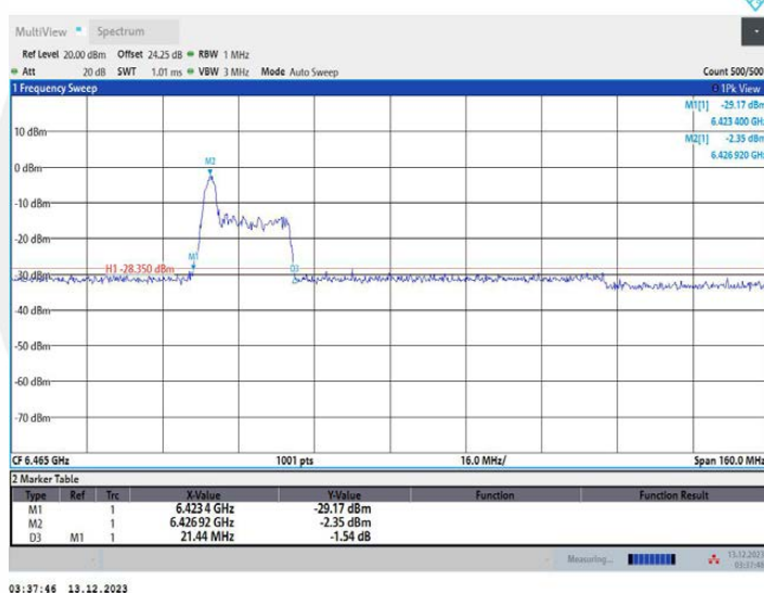
11AX80MIMO_Ant1_6465_52Tone_RU37
