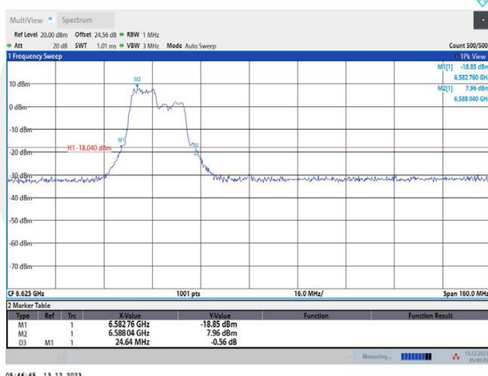
11AX80MIMO_Ant1_6625_242Tone_RU61
