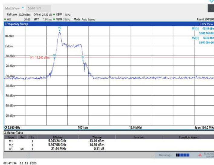
11AX80MIMO_Ant1_5985_52Tone_RU37
