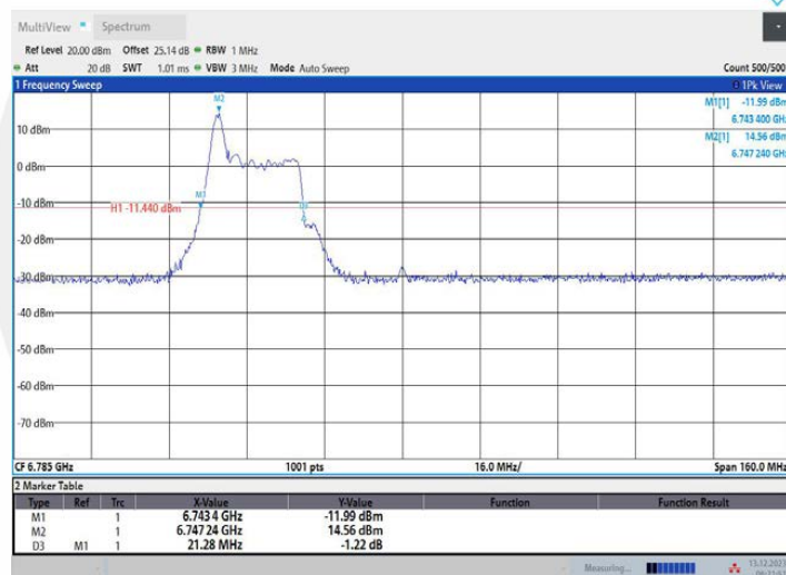
11AX80MIMO_Ant1_6785_52Tone_RU37
