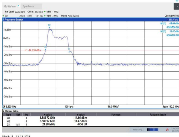
11AX80MIMO_Ant1_6625_106Tone_RU53
