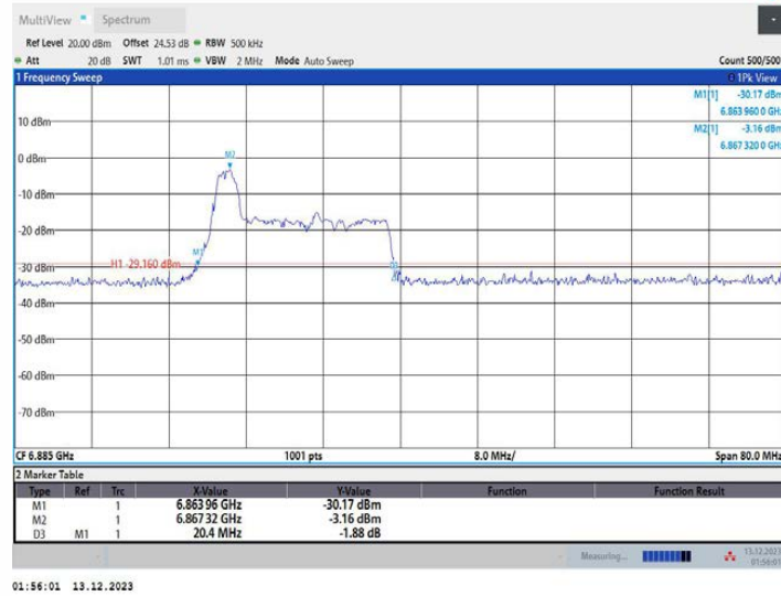
11AX40MIMO_Ant2_6885_52Tone_RU37
