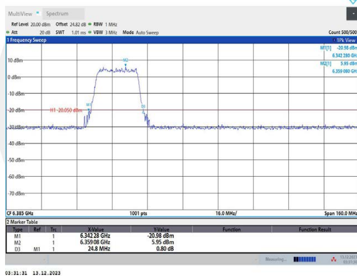
11AX80MIMO_Ant2_6385_484Tone_RU65
