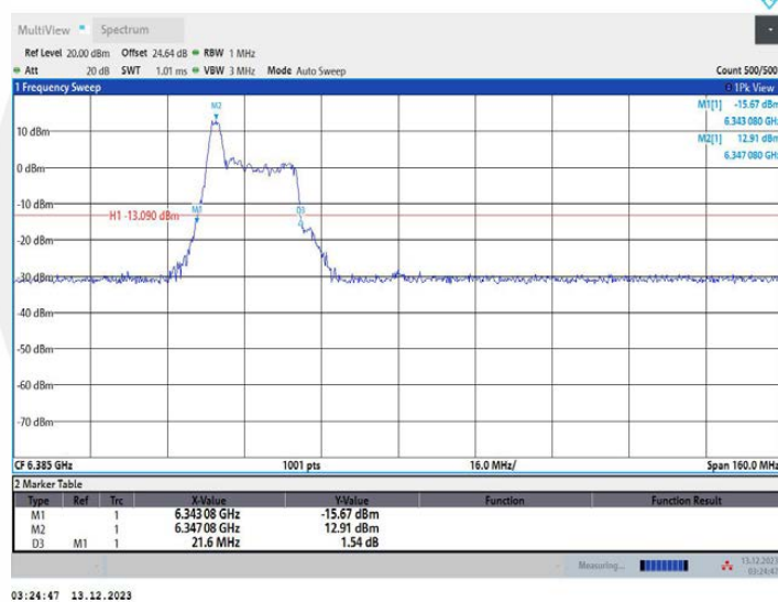
11AX80MIMO_Ant1_6385_52Tone_RU37
