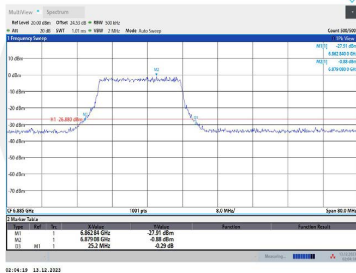
11AX40MIMO_Ant1_6885_26Tone_RU0
