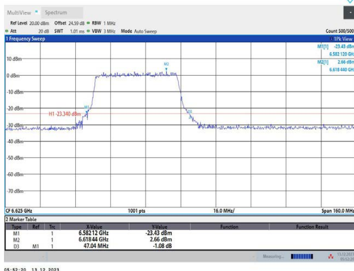
11AX80MIMO_Ant1_6625_26Tone_RU0
